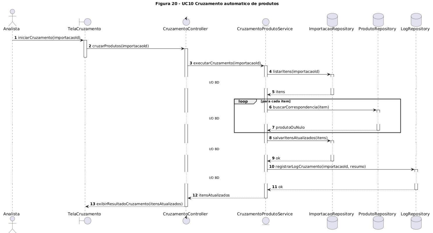
Figura 20. Diagrama de sequência de projeto – UC10
