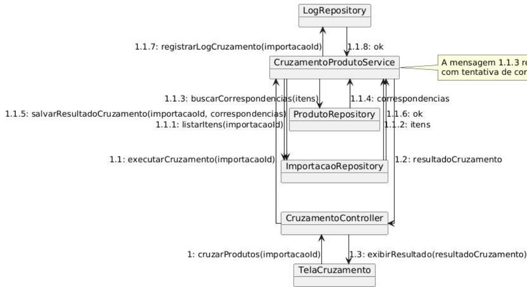
Figura 26 - Diagrama de comunicacao (UC10)
