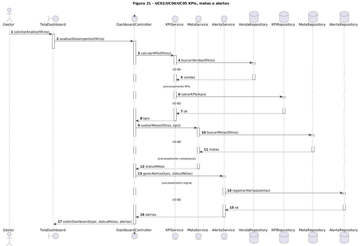
Figura 21. Diagrama de sequência de projeto – UC02/UC04/UC05
