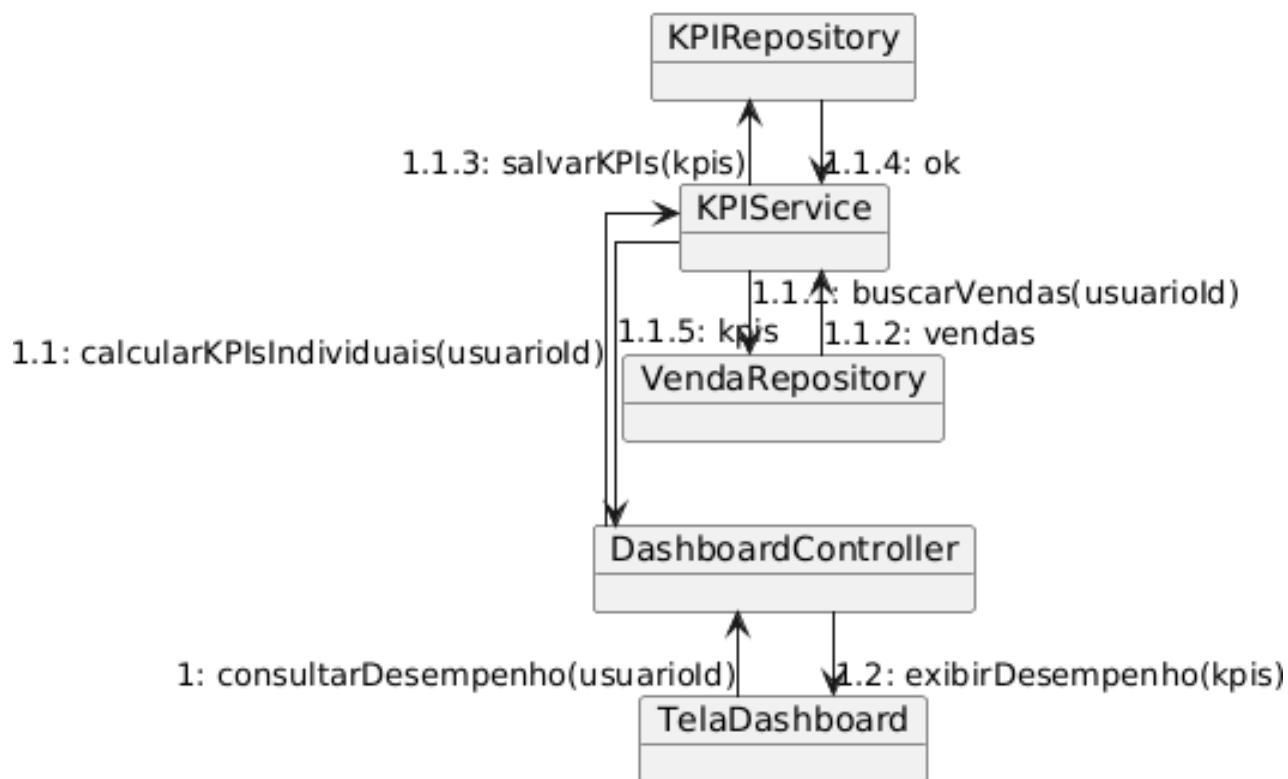
Figura 24. Diagrama de comunicação – UC01
