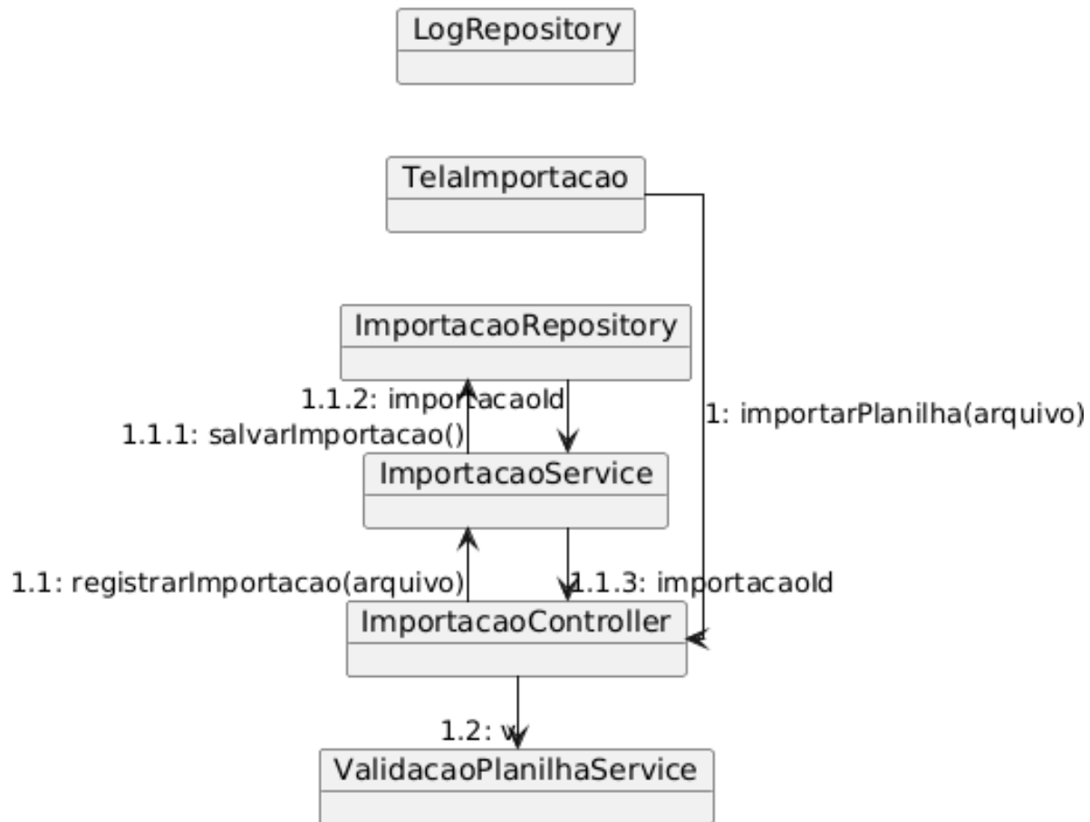
Figura 25. Diagrama de comunicação – UC08/UC09/UC11
