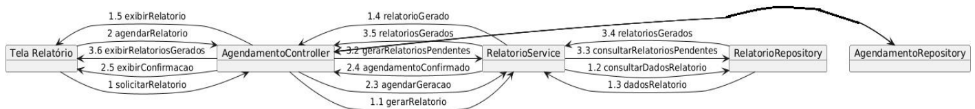
Figura 28 - Diagrama de Comunicação (UC06/UC07/UC15)
