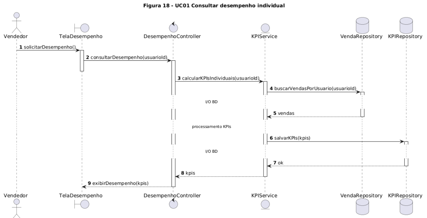
Figura 18. Diagrama de sequência de projeto UCI
