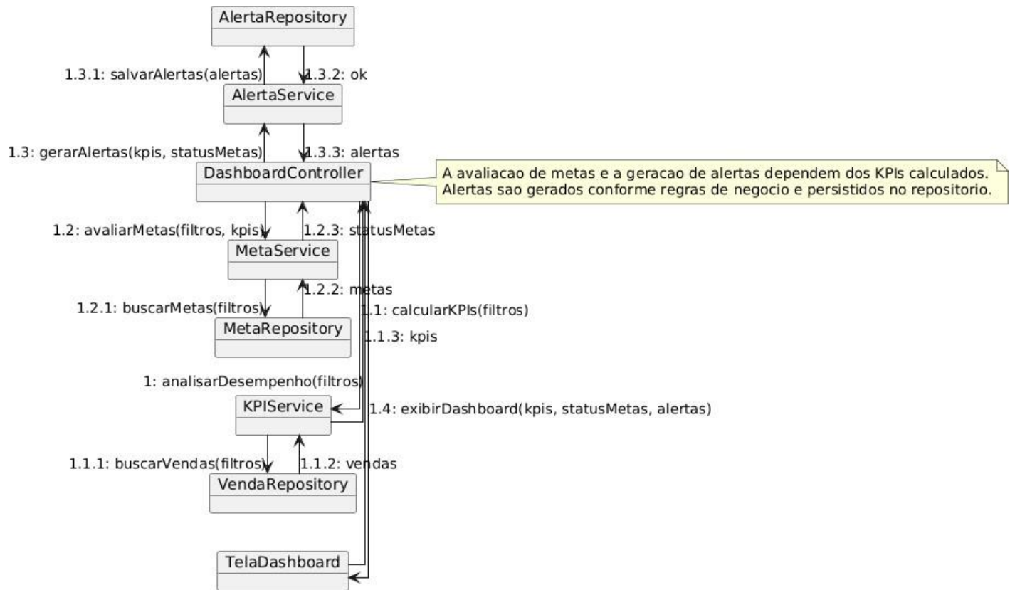
Figura 27 - Diagrama de comunicacao (UC02/UC04/UC05)
