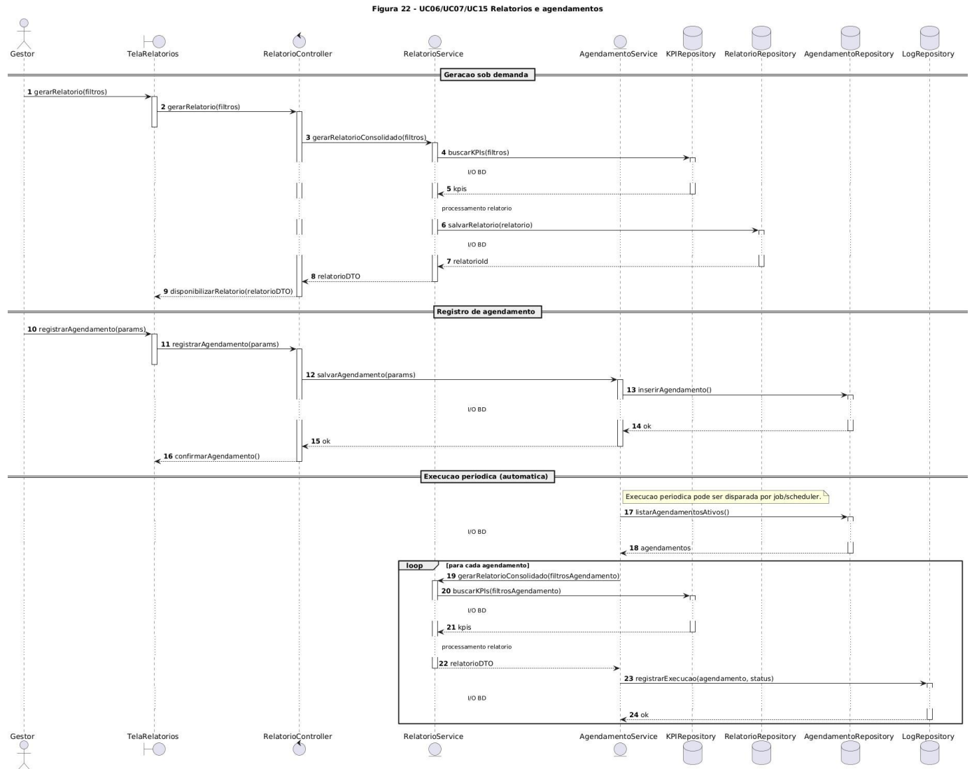
Figura 22. Diagrama de sequência de projeto – UC06/UC07/UC15
