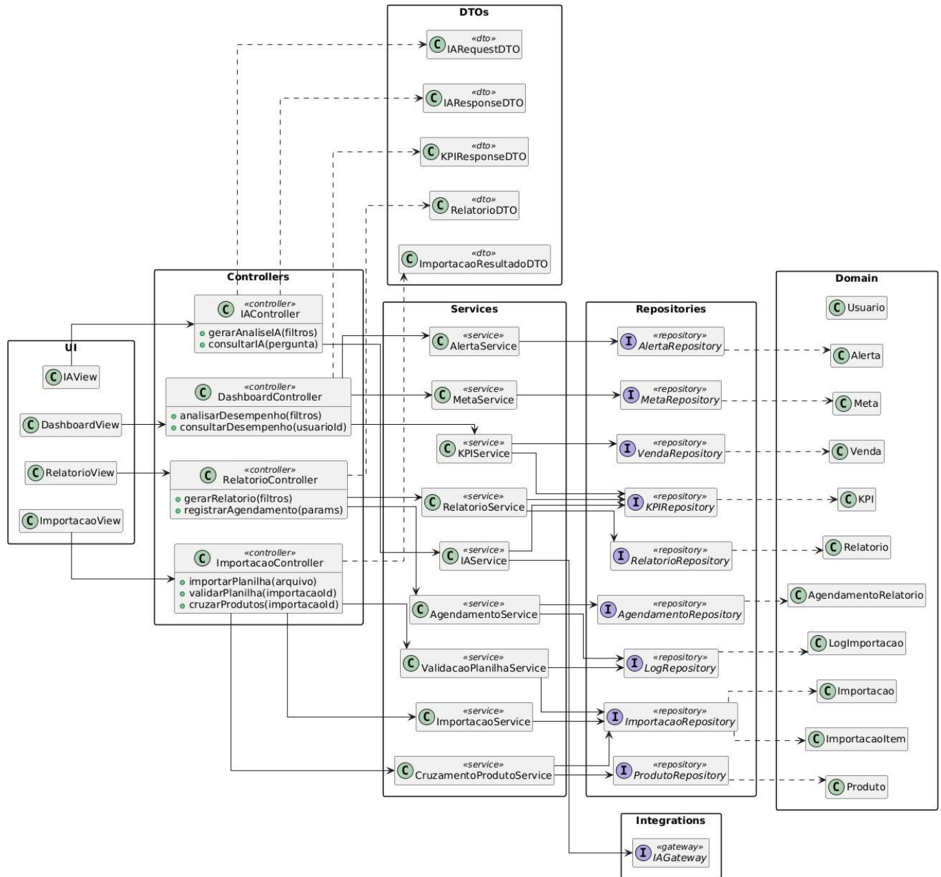
Figura 31. Persistência da arquitetura
