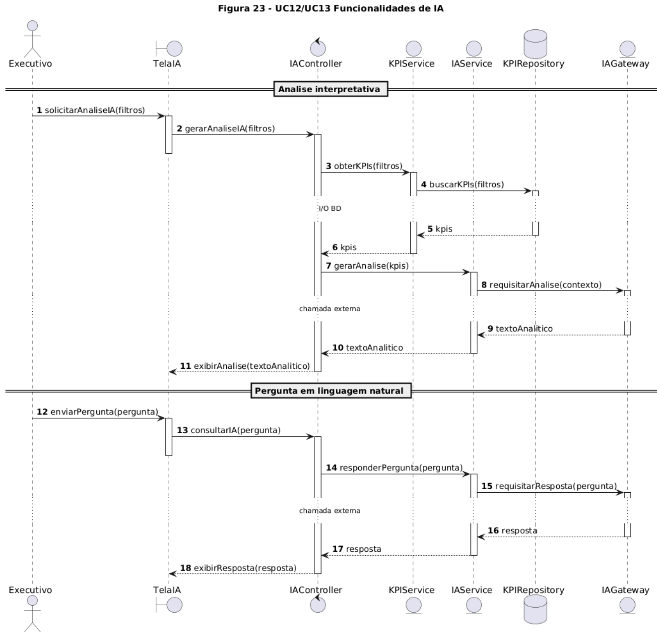
Figura 23. Diagrama de sequência de projeto – UC12/UC13
