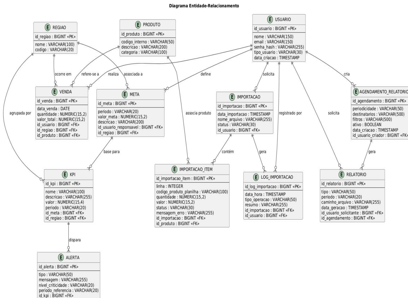
Figura 45. Diagrama Entidade Relacionamento
