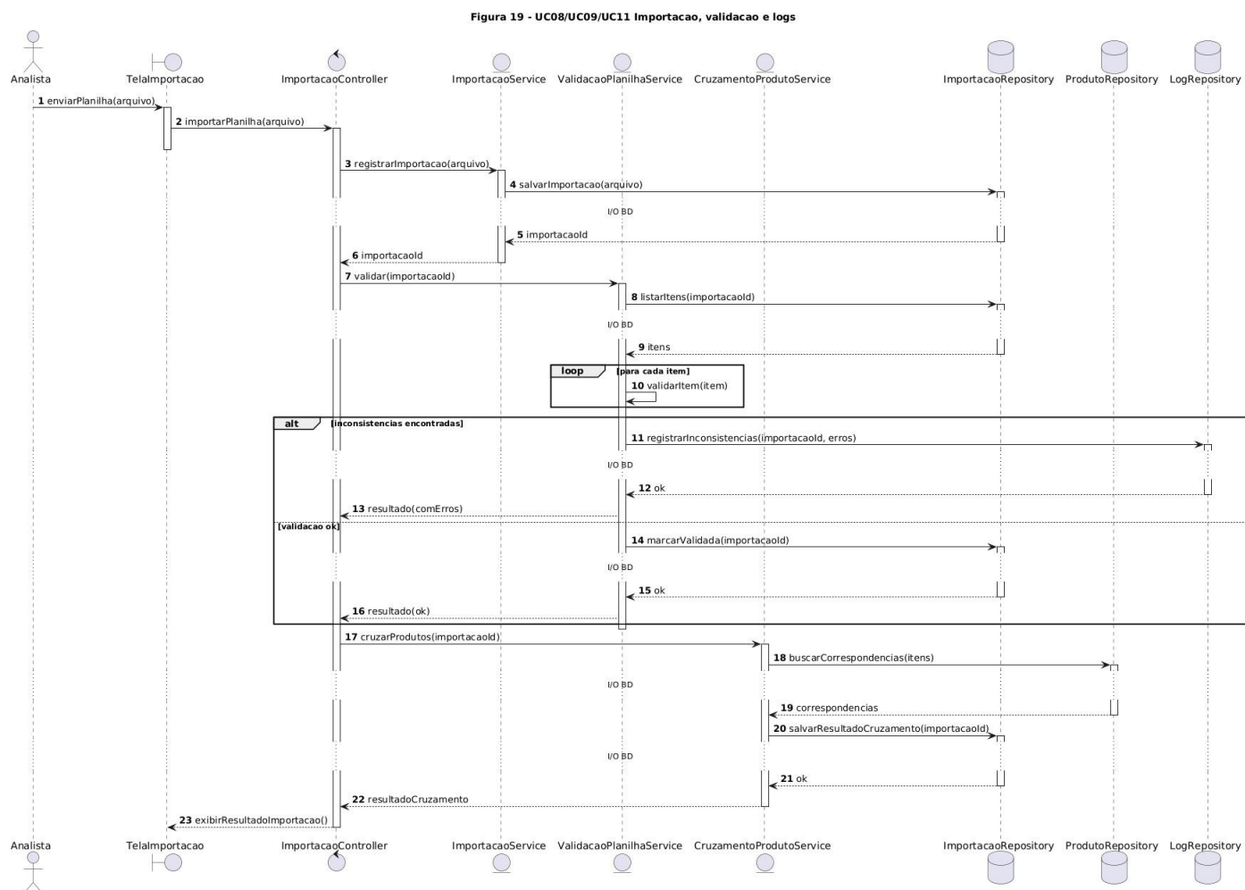
Figura 19. Diagrama de sequência de projeto – UC08/UC09/UC11
