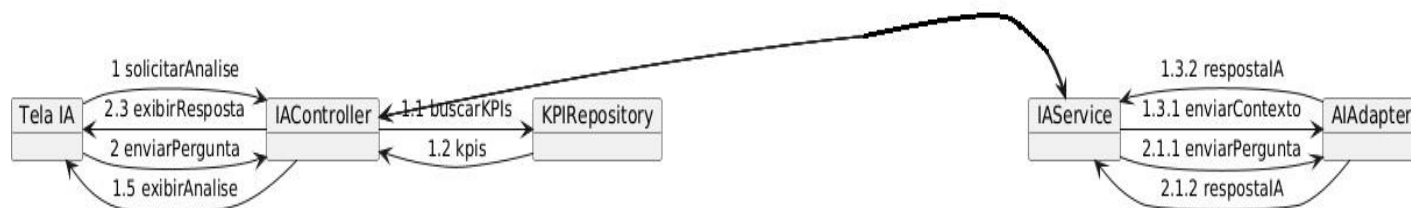
Figura 29 - Diagrama de Comunicação (UC12 / UC13)
