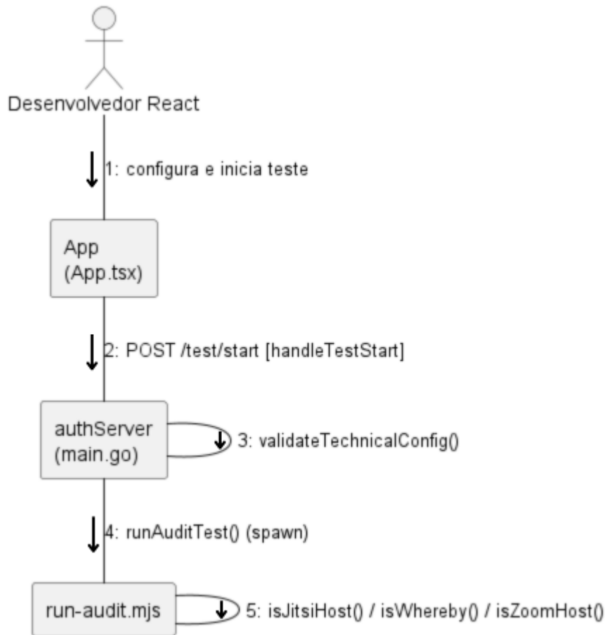
Figura 13: Diagrama de Comunicação de Configuração e Validação
