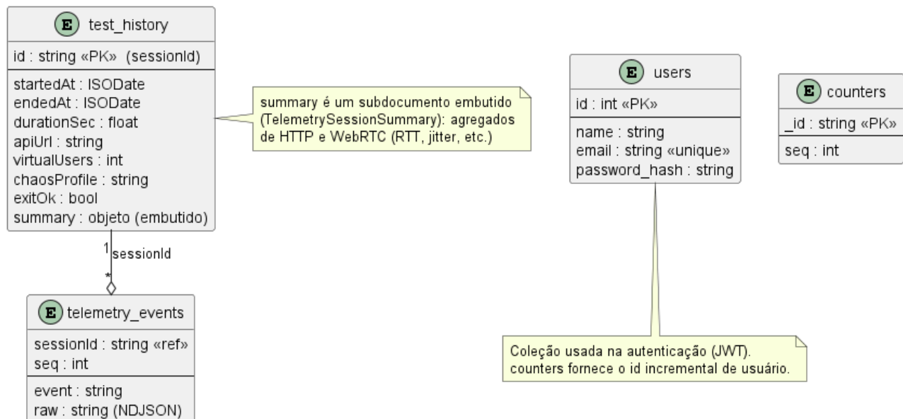
Figura 33: Diagrama de Entidade e Relacionamento
