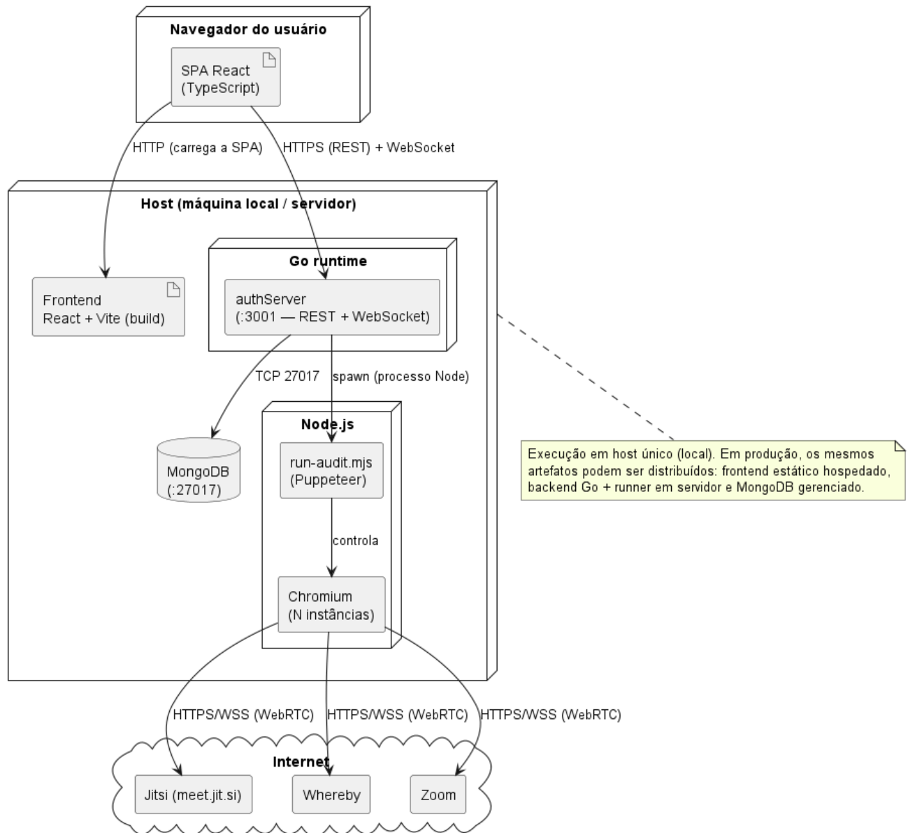
Figura 19: Diagrama de Implantação
