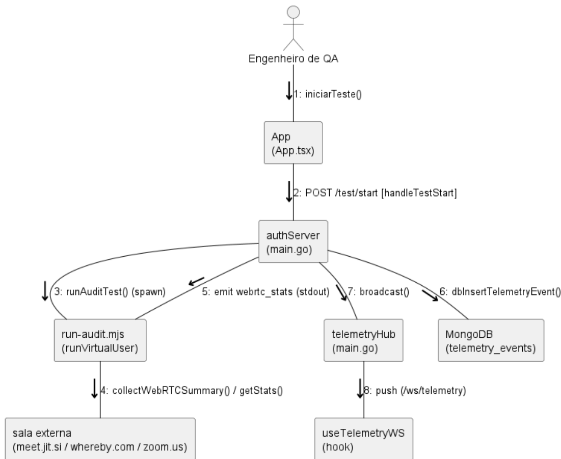
Figura 14: Diagrama de Comunicação de Execução e Telemetria
