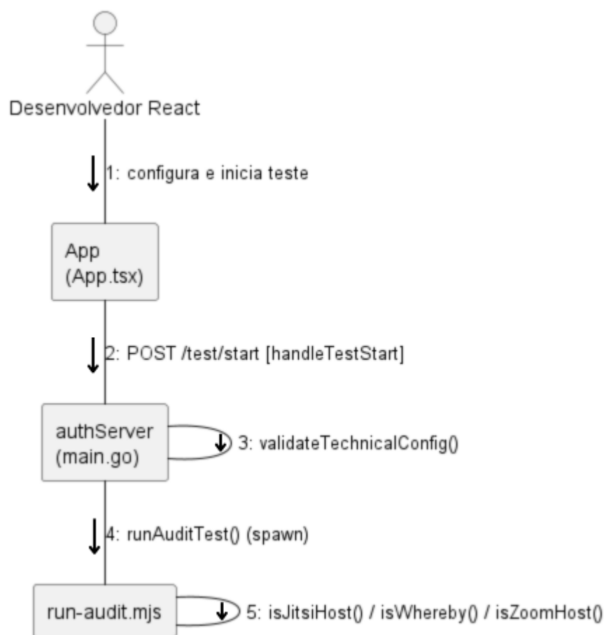
Figura 13: Diagrama de Comunicação de Configuração e Validação
