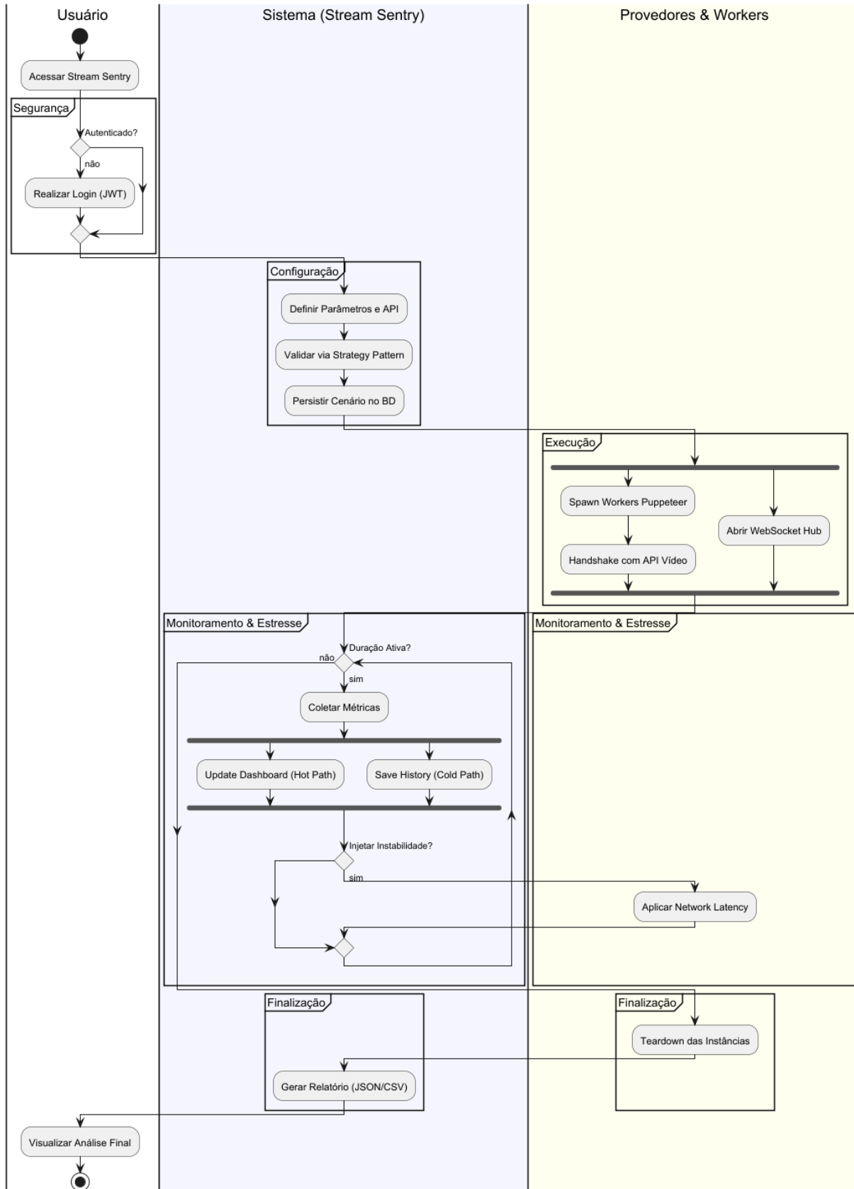
Figura 17: Diagrama de Atividade
