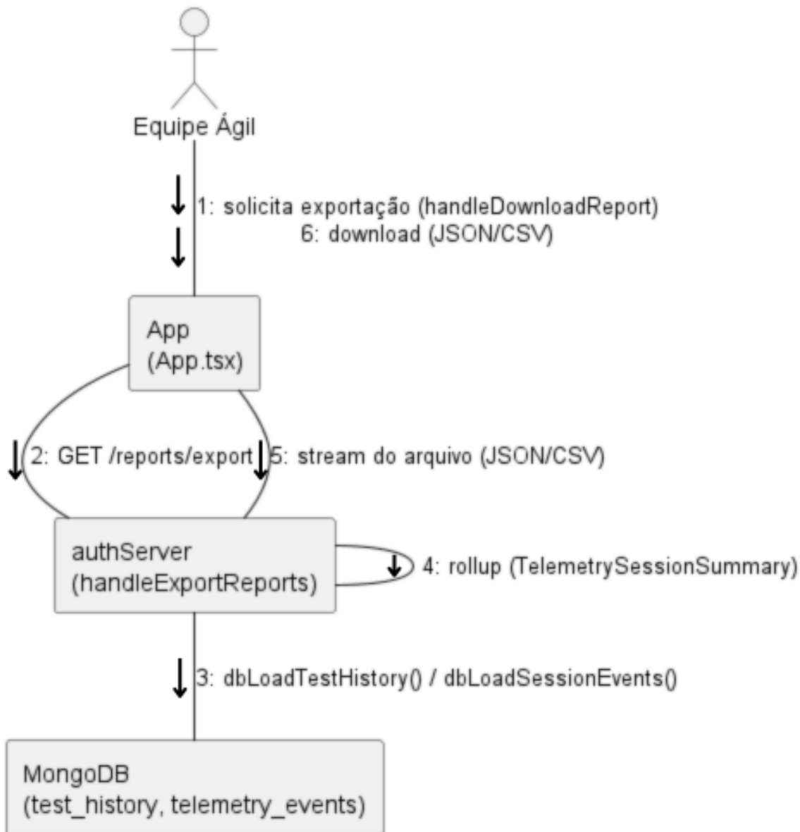
Figura 15: Diagrama de Comunicação de Consolidação de Relatório
