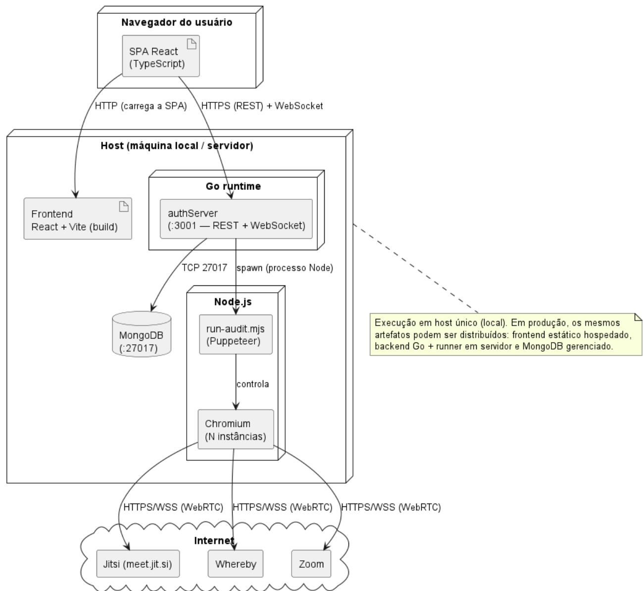
Figura 17: Diagrama de Implantação
