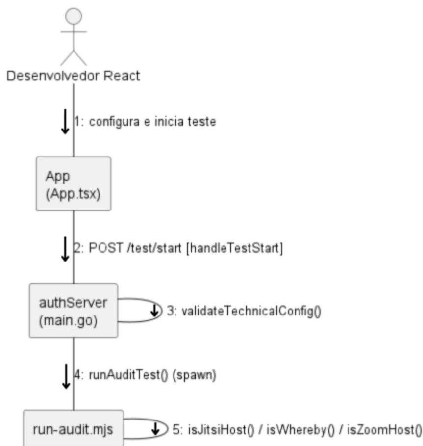
Figura 15: Diagrama de Comunicação de Configuração e Validação
