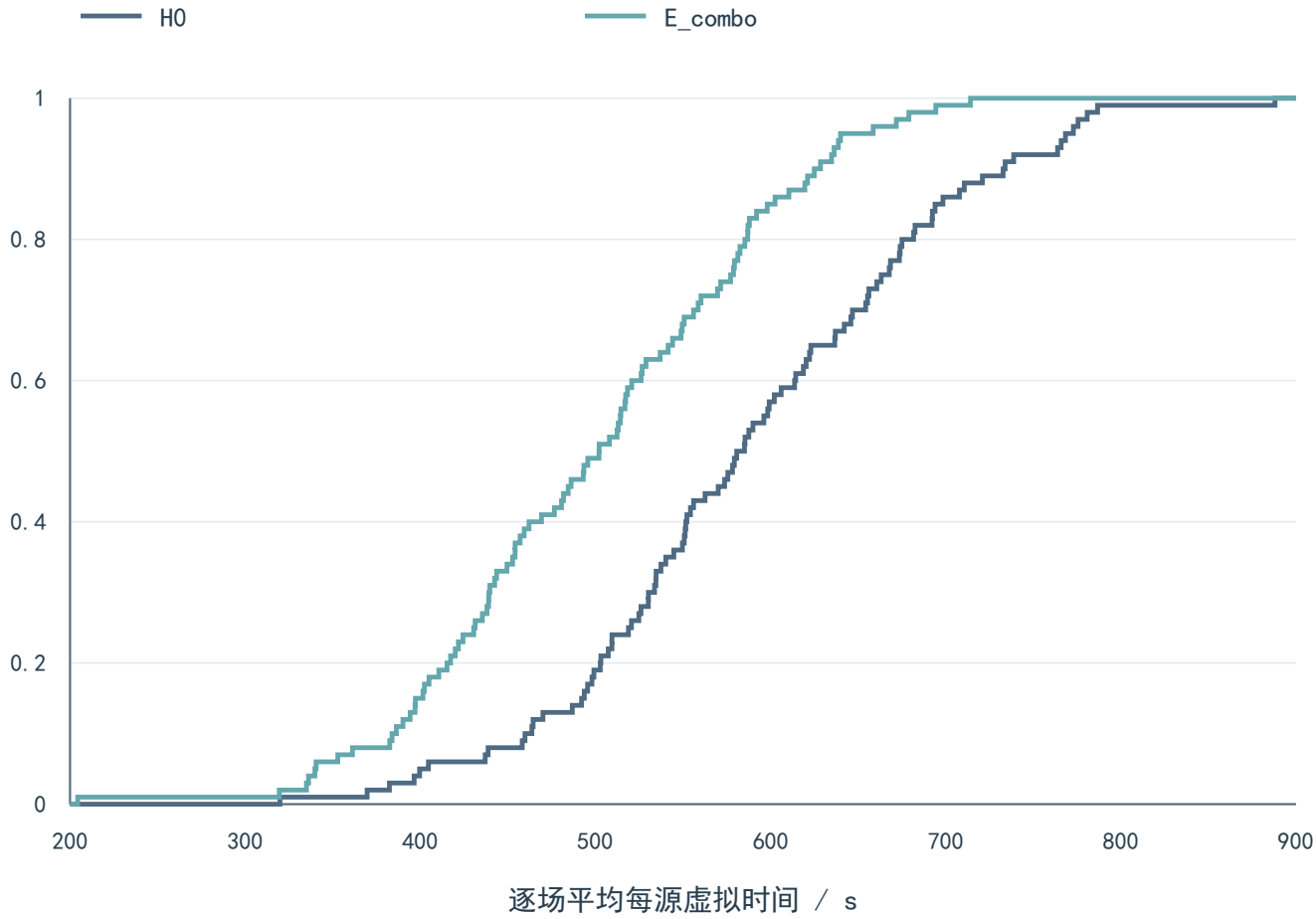
经验累积分布
