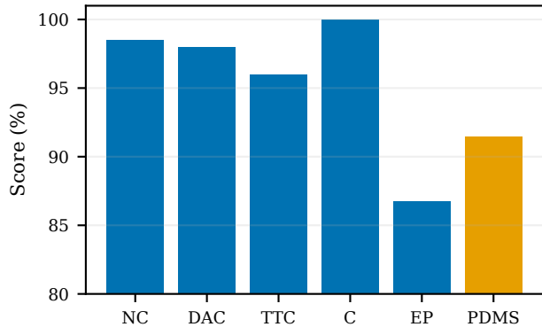
NAVSIM v1
