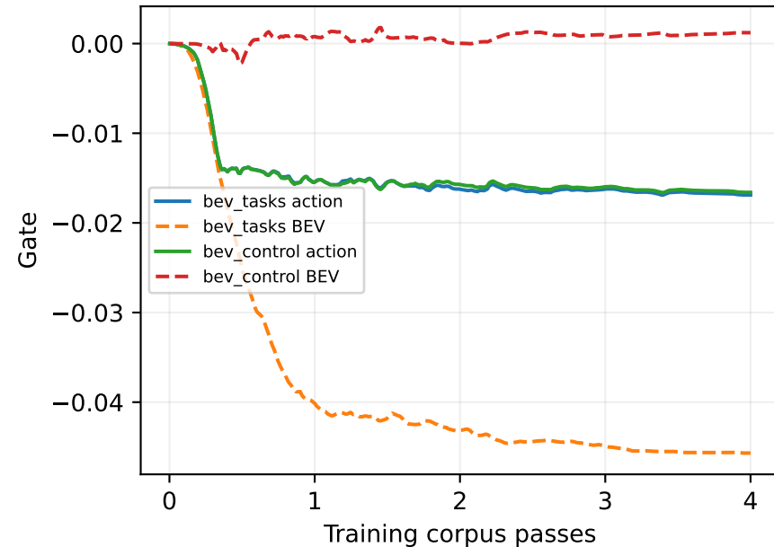
Learned gates, actual values
