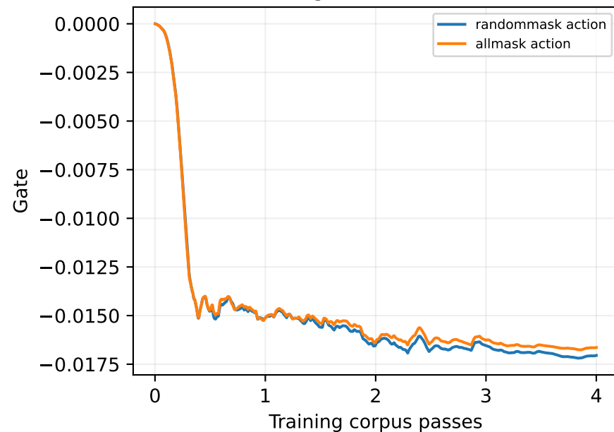
Learned gates, actual values
