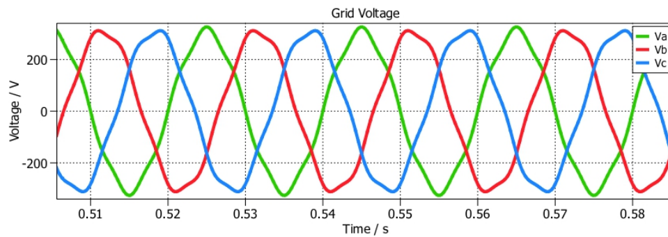
Figura 1: Voltaje de la red eléctrica con desbalances y armónicos.
