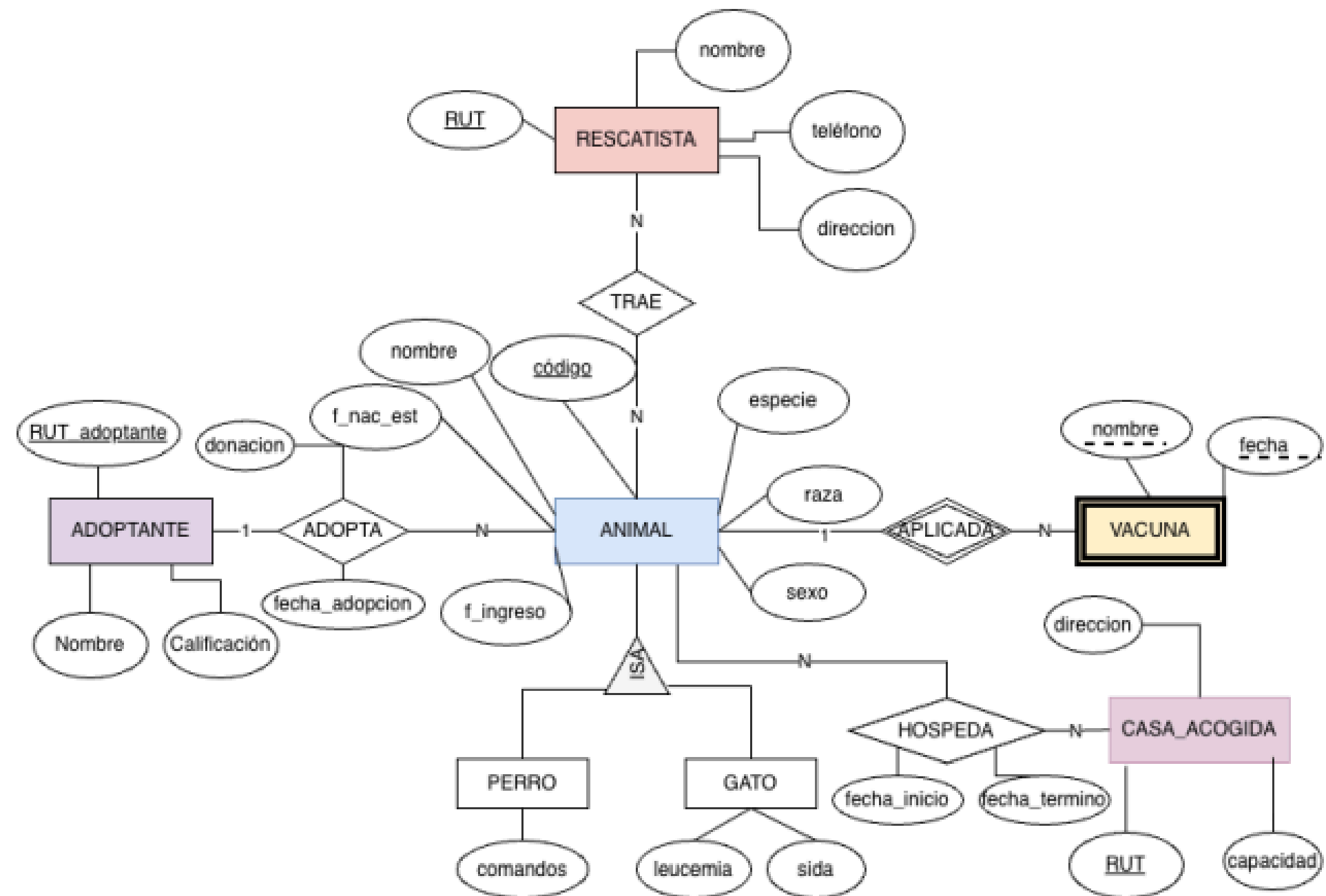
Figura 1: Diagrama Entidad Relación
