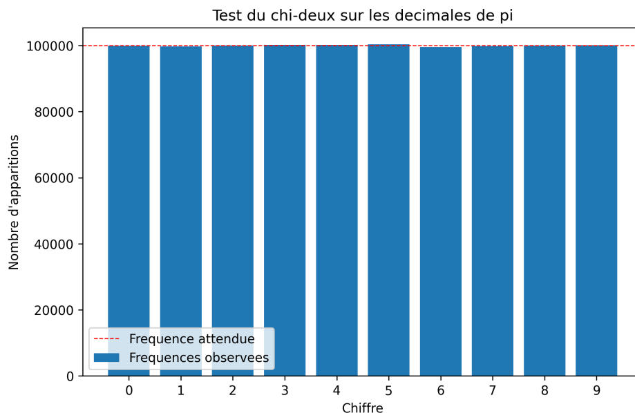
FIGURE 1 – Fréquences observées des chiffres de \pi et fréquence attendue sous uniformité.
