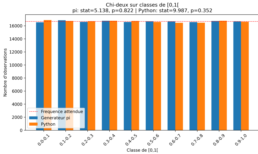
FIGURE 5 – Comparaison des deux générateurs par test du \chi^2 sur dix classes de [0, 1[ .
