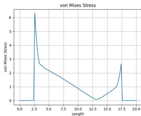
図 14 \rho = 1 における応力分布
