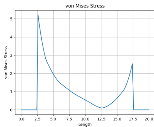
図 16 \rho = 4 における応力分布
