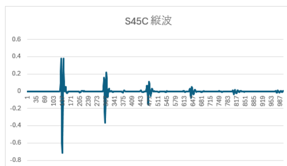
図 2 S45C 縦波
