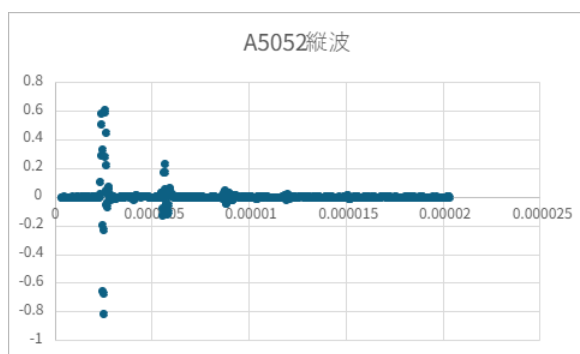
図 3 A5052 縦波
