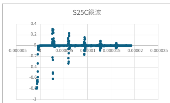
図 1 S25C 縦波
