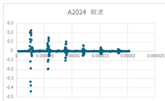
図 4 A2024 縦波
