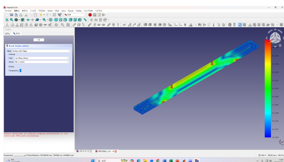
図 24 \rho = 1 における応力分布（中程度）
