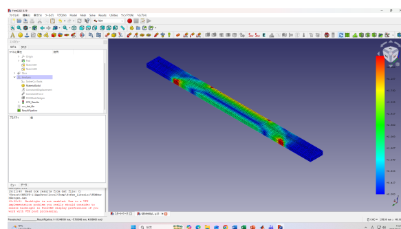
図 25 \rho = 1 における応力分布（細かい）
