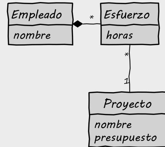
Ejemplo clase asociación con composición
