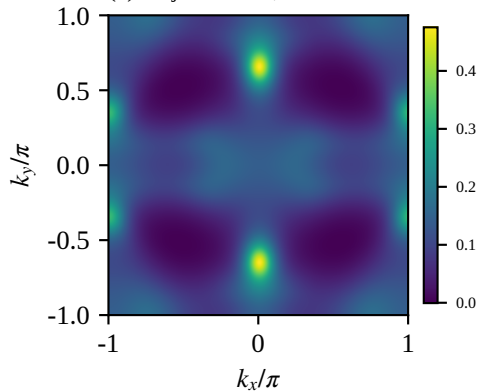
(d) Projected term, \varepsilon=6/5
