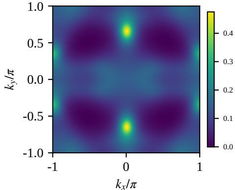
(d) Projected term, \varepsilon = 1.2
