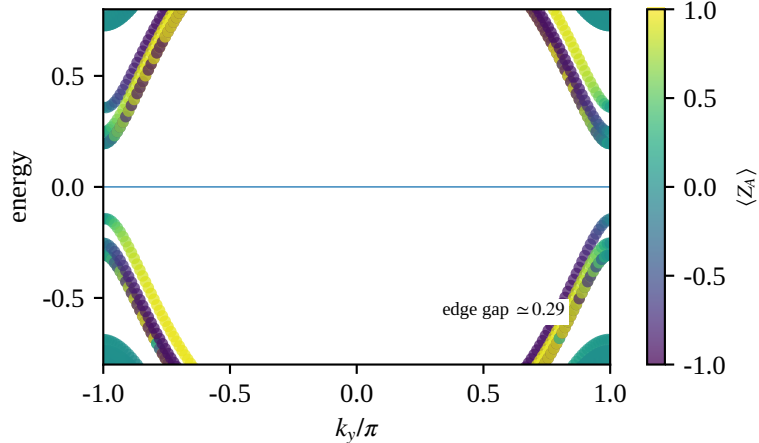
(d) Pump window
