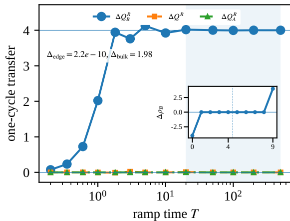
(d) Pump window
