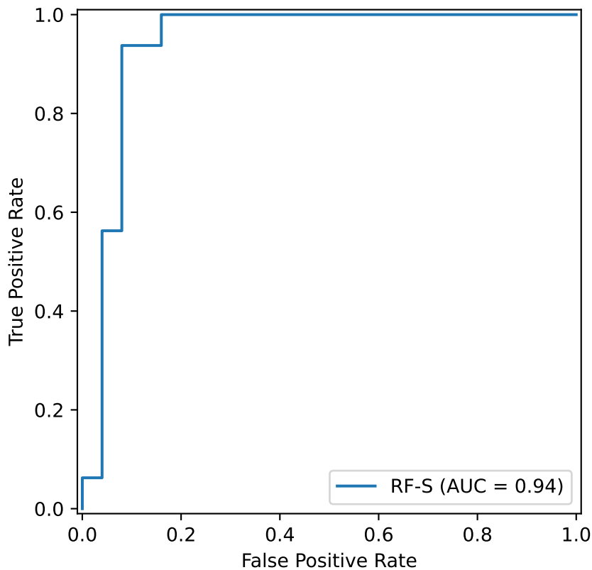
ROC - Tobramycin_AB (Class S)
