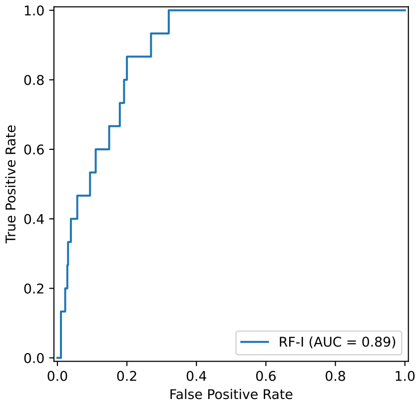
ROC - Meropenem_AB (Class I)
