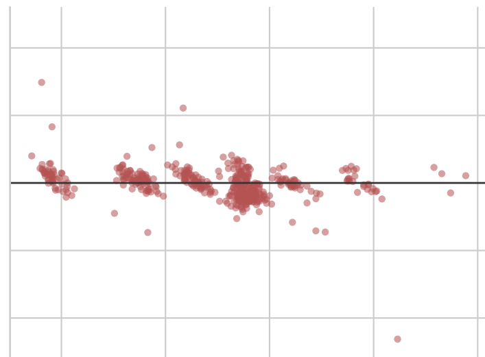
FPCR
