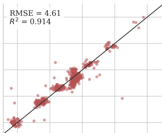
FPCR
