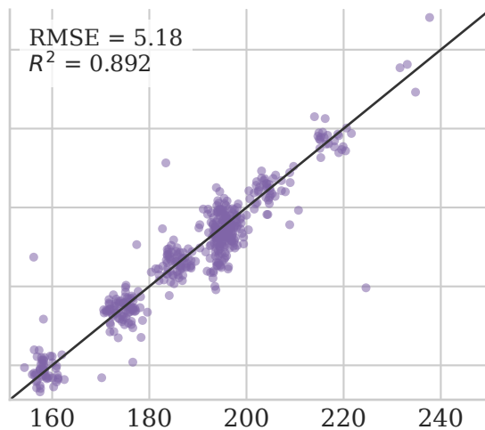
FPCR
