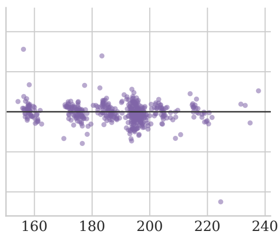
FPCR
