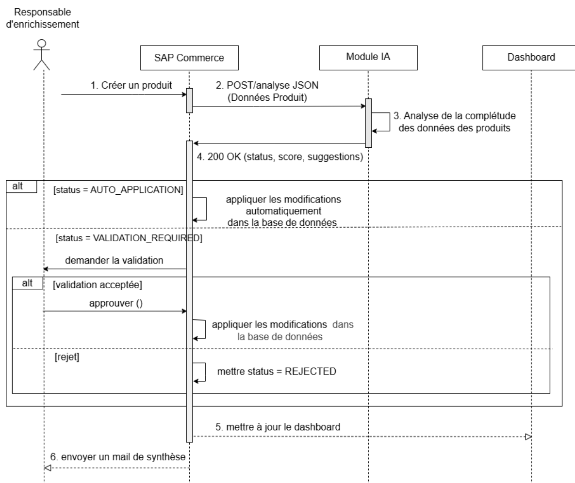
FIGURE 4.6 – Diagramme de séquence global de l'interaction utilisateur et des processus système
