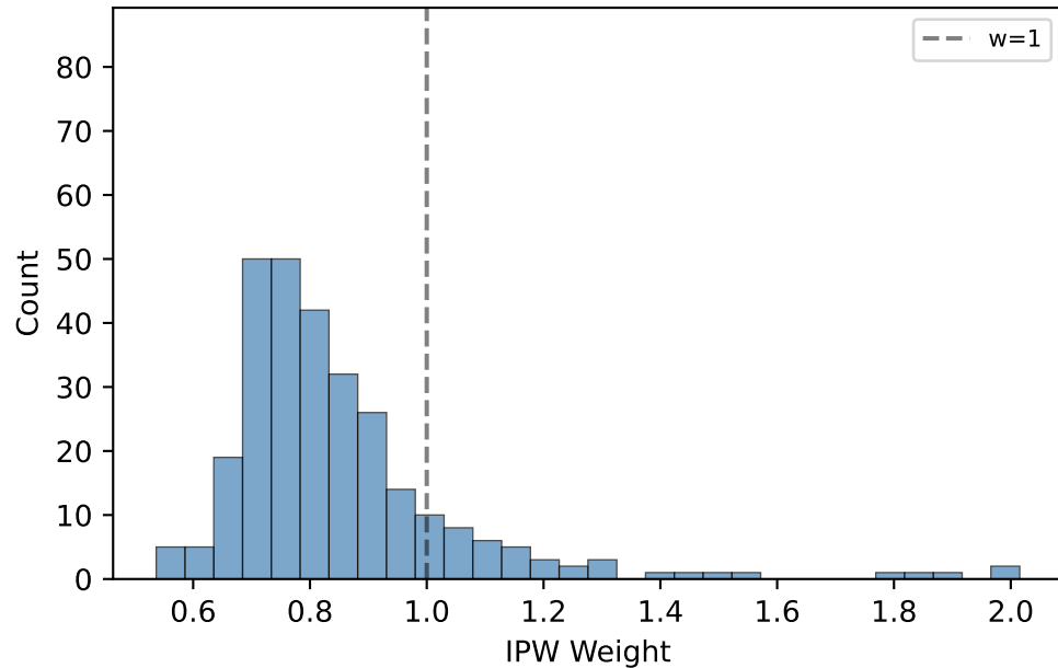
NGC (N=289, ESS=272)
