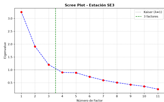
Figura 12: Scree plot de la estación SE3 (Cadereyta) con el criterio de Kaiser ( \lambda = 1 ) y el número de factores retenidos.
