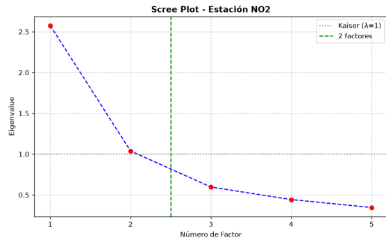
Figura 11: Scree plot de la estación NO2 (García) con el criterio de Kaiser ( \lambda = 1 ) y el número de factores retenidos.
