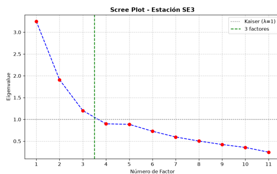
Figure 12: Scree plot de la estación SE3 (Cadereyta) con el criterio de Kaiser ( \lambda = 1 ) y el número de factores retenidos.
