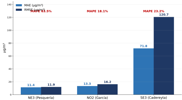
Figure 17: Comparativa de métricas de error (MAE, RMSE y MAPE) obtenidas en la ventana de validación fuera de muestra (7 horas) para las tres estaciones.
