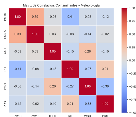
Figure 3: Matriz de correlación entre los contaminantes y las variables meteorológicas retenidas ( PM_{10} , PM_{2.5} , TOUT , RH , WSR , PRS ). La marcada interdependencia entre predictores justifica la reducción de dimensionalidad mediante el AFE.
