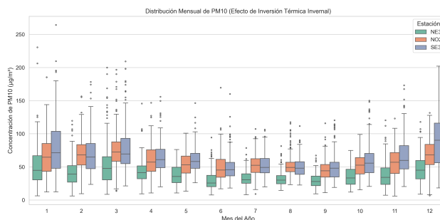
Figure 2: Distribución mensual de PM_{10} para el triplete representativo (2020–2025). La elevación de las medianas durante los meses de invierno evidencia el efecto de las inversiones térmicas sobre la acumulación de contaminantes.
