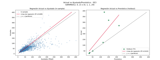
Figure 7: Pronóstico horario fuera de muestra (horizonte de 7 horas) vs valores reales de PM_{10} en SE3 (Cadereyta).
