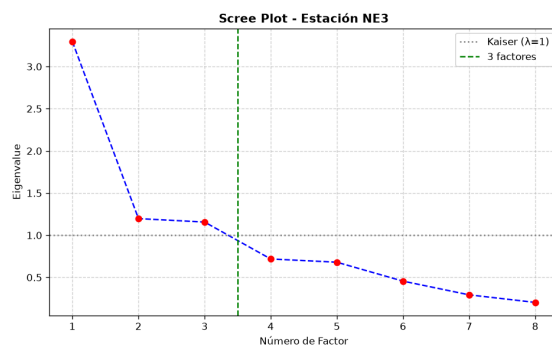
Figure 13: Scree plot de la estación NE3 (Pesquería) con el criterio de Kaiser ( \lambda = 1 ) y el número de factores retenidos.
