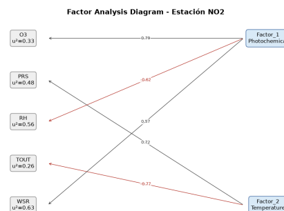
Figure 14: Diagrama de cargas factoriales de la estación NO2 (García). El grosor de la flecha es proporcional a la carga y el color rojo indica carga negativa.
