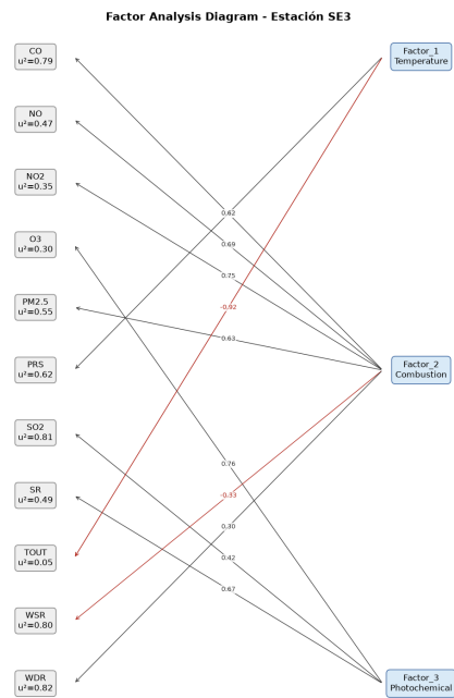
Figure 15: Diagrama de cargas factoriales de la estación SE3 (Cadereyta). El grosor de la flecha es proporcional a la carga y el color rojo indica carga negativa.
