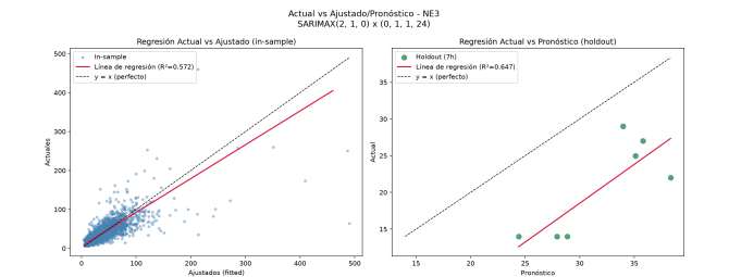
Figure 8: Pronóstico horario fuera de muestra (horizonte de 7 horas) vs valores reales de PM_{10} en NE3 (Pesquería).
