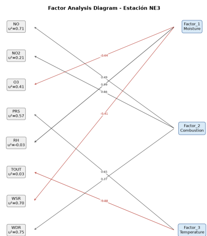
Figure 16: Diagrama de cargas factoriales de la estación NE3 (Pesquería). El grosor de la flecha es proporcional a la carga y el color rojo indica carga negativa.
