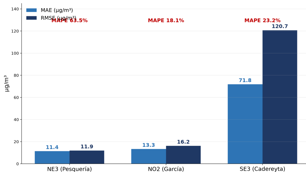
Figura 17: Comparativa de métricas de error (MAE, RMSE y MAPE) obtenidas en la ventana de validación fuera de muestra (7 horas) para las tres estaciones.
