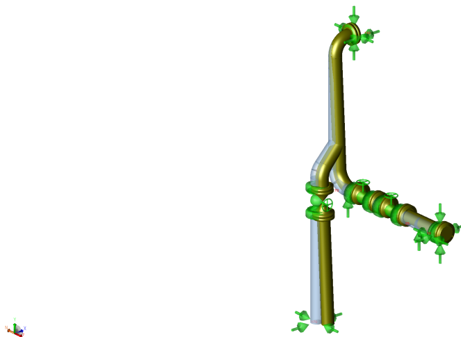
Figura 3: Configuración deformada del modelo superpuesta a la geometría original (CAESAR II, job P2603-PR-SIM-002).
