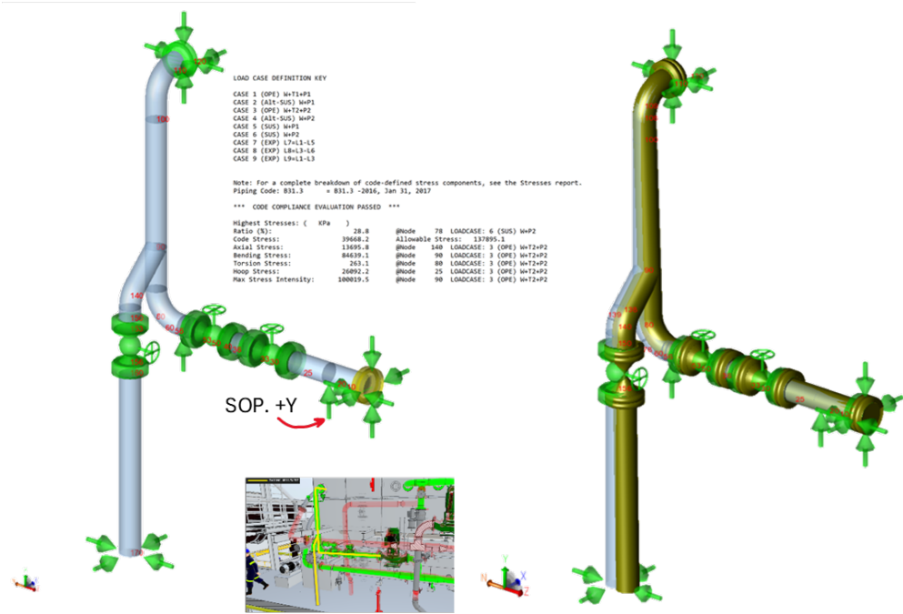
DESCARGA DE BOMBA DE RECIRCULACION 1 DDW
