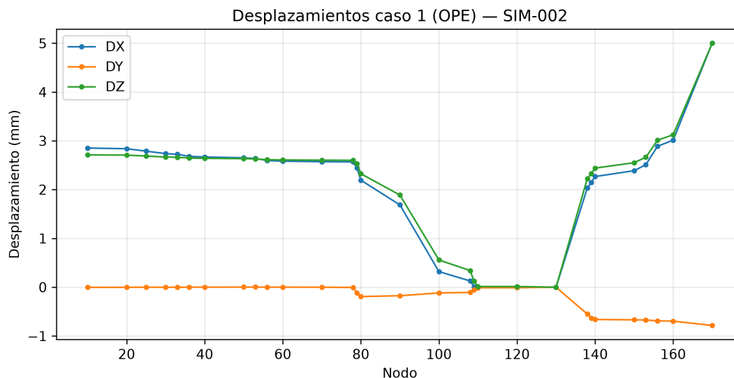
Figura 3: Perfil de desplazamientos nodales DX , DY y DZ en el caso 1 (OPE) W+T1+P1.
