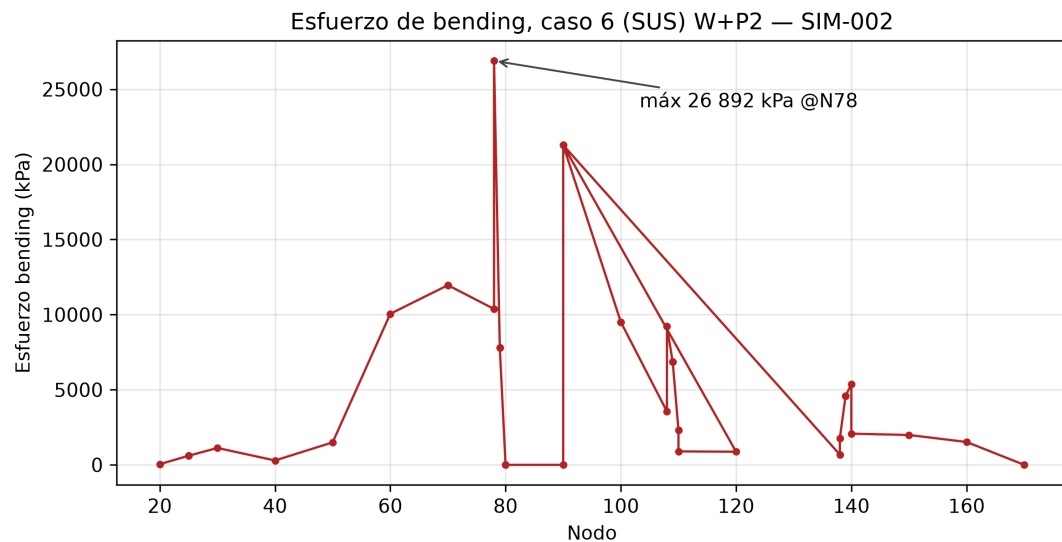
Figura 4: Perfil de esfuerzo de flexión por nodo, caso crítico 6 (SUS) W+P2. Máximo: 26 891,5 kPa en el nodo 78.
