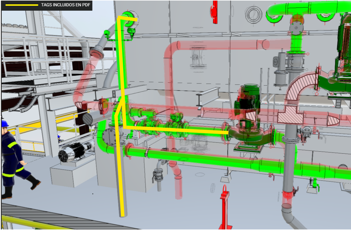
Figura 1: Vista del modelo 3D de la línea de descarga de la bomba de recirculación 1 DDW (PCF103, AutoCAD Plant 3D 2027).
