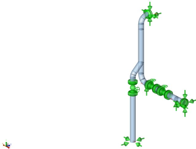
Figura 2: Modelo de CAESAR II con la numeración de nodos y los soportes y restricciones de la línea (job P2603-PR-SIM-002).
