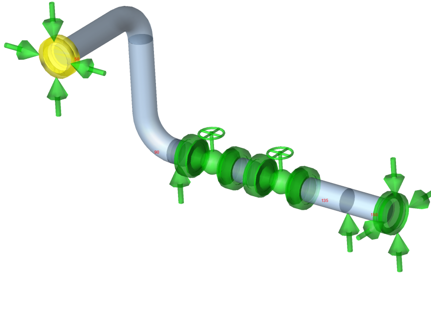
Figura 7: Modelo de CAESAR II con los soportes y restricciones de la línea, vista 2 (job P2603-PR-SIM-003).
