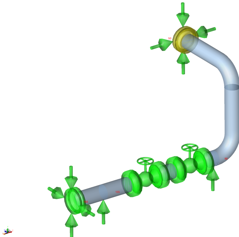
Figura 6: Modelo de CAESAR II con los soportes y restricciones de la línea, vista 1 (job P2603-PR-SIM-003).
