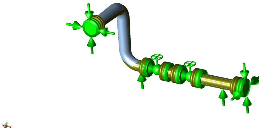
Figura 3: Modelo de CAESAR II con la forma deformada de la línea en condición de operación; los desplazamientos se representan amplificados con fines de visualización (job P2603-PR-SIM-003).
