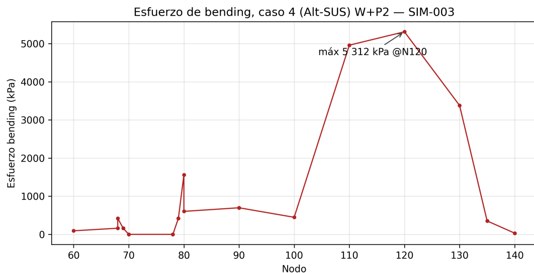
Figura 4: Perfil de esfuerzo de flexión por nodo, caso crítico 4 (Alt-SUS) W+P2. Máximo: 5312,4 kPa en el nodo 120.
