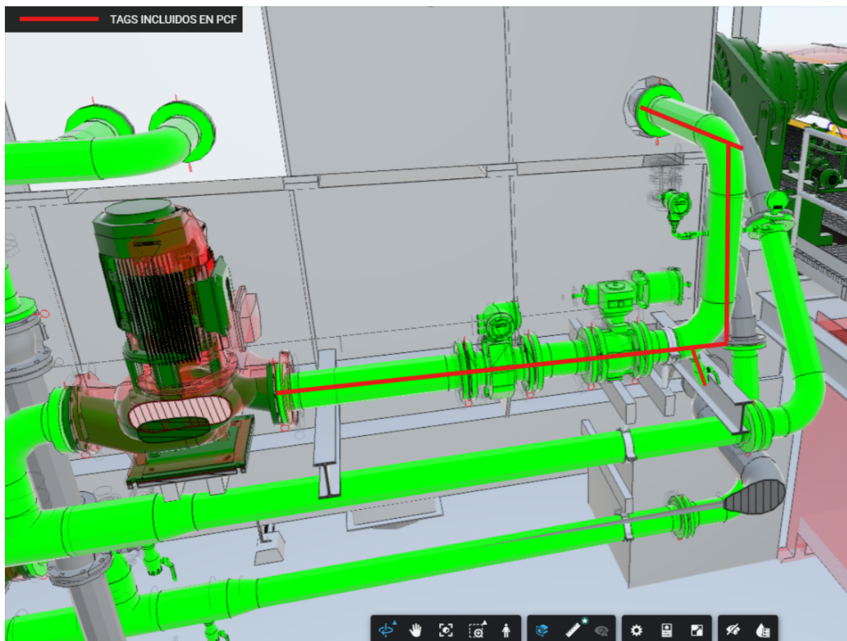
Figura 1: Isométrico de la línea de descarga de la bomba de recirculación 2 DDW (PCF104, AutoCAD Plant 3D 2027).
