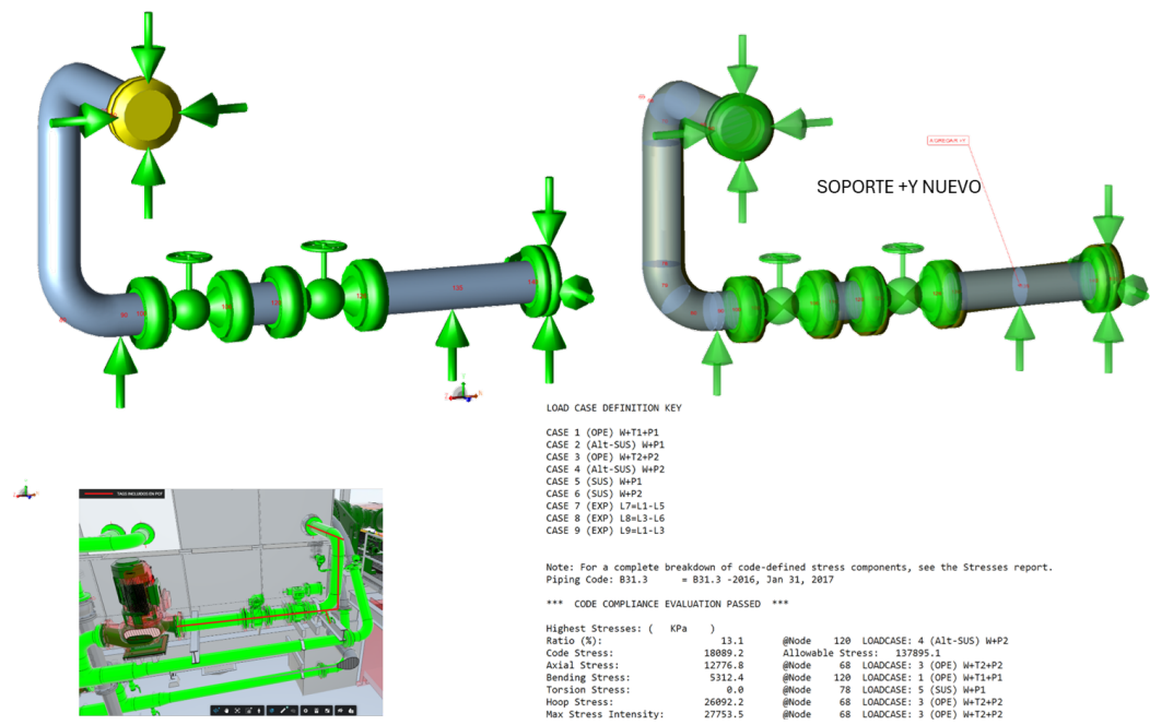
Figura A.4: Resultados gráficos del modelo: vistas del sistema y salida de CAESAR II.
