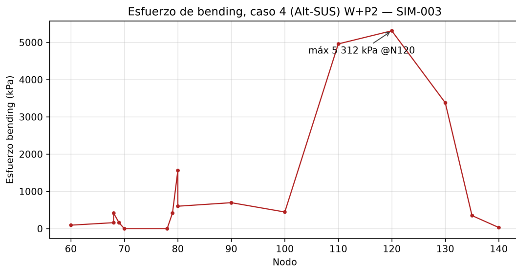
Figura 3: Perfil de esfuerzo de flexión por nodo, caso crítico 4 (Alt-SUS) W+P2. Máximo: 5312,4 kPa en el nodo 120.
