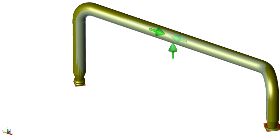
Figura 3: Vista del modelo de CAESAR II con la posición deformada de la línea (job P2603-PR-SIM-007).
