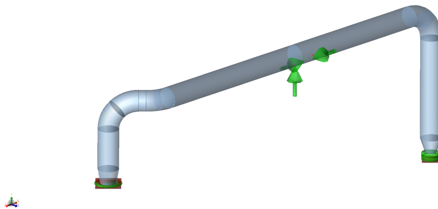
Figura 6: Modelo de CAESAR II con los soportes y restricciones de la línea: anclas en los nodos 10 y 110, y soporte rígido vertical (+Y) con guía axial en el nodo 75 (job P2603-PR-SIM-007).
