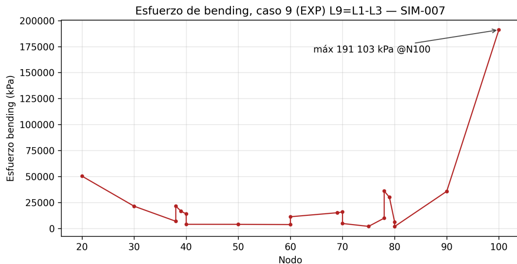
Figura 4: Perfil de esfuerzo de flexión por nodo, caso crítico 9 (EXP) L9=L1-L3. Máximo: 191 102,8 kPa en el nodo 100.
