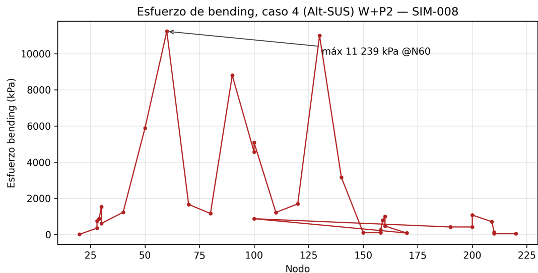
Figura 4: Perfil de esfuerzo de flexión por nodo, caso crítico 4 (Alt-SUS) W+P2. Máximo: 11 239,1 kPa en el nodo 60.
