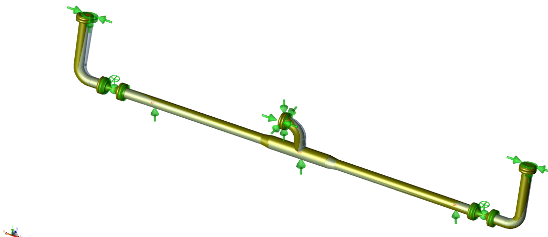
Figura 3: Vista del modelo de CAESAR II con la geometría deformada de la línea superpuesta a su posición inicial (job P2603-PR-SIM-008).
