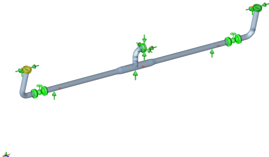
Figura 6: Modelo de CAESAR II con los soportes y restricciones de la línea (job P2603-PR-SIM-008).
