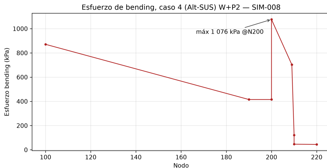
Figura 3: Perfil de esfuerzo de flexión por nodo, caso crítico 4 (Alt-SUS) W+P2. Máximo: 1076,3 kPa en el nodo 200.
