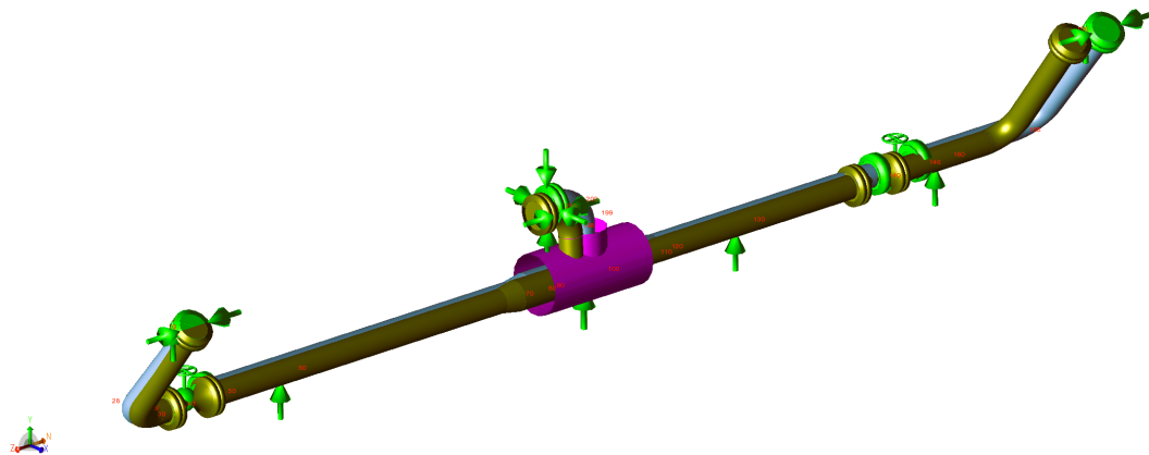
Figura 3: Modelo de CAESAR II con la posición inicial y la posición desplazada de la línea en la condición de desplazamientos máximos (job P2603-PR-SIM-009).
