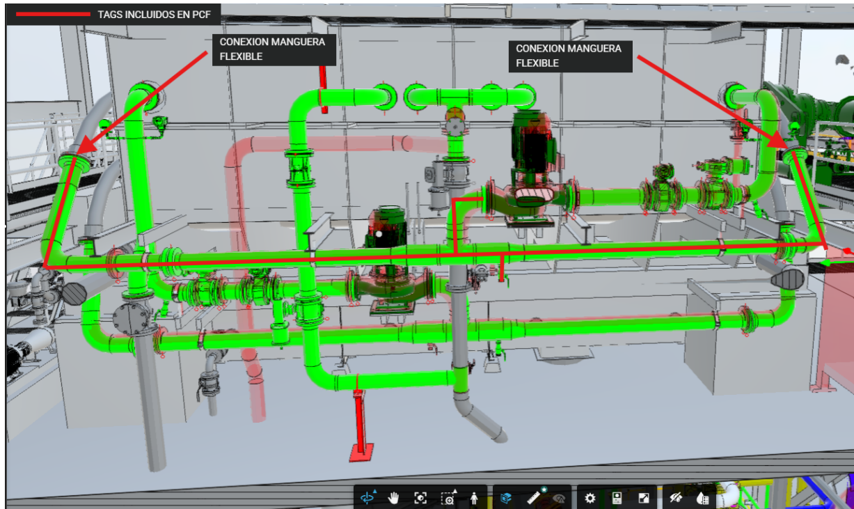
Figura 1: Isométrico de la línea de succión de la bomba de recirculación 2 DDW (PCF105, AutoCAD Plant 3D 2027).
