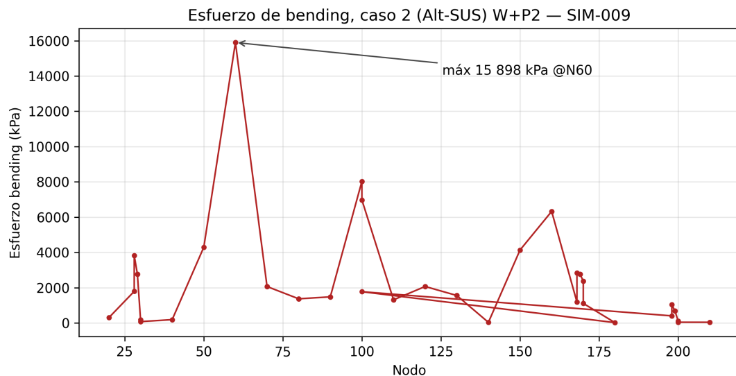
Figura 4: Perfil de esfuerzo de flexión por nodo, caso crítico 2 (Alt-SUS) W+P2. Máximo: 15 898,0 kPa en el nodo 60.
