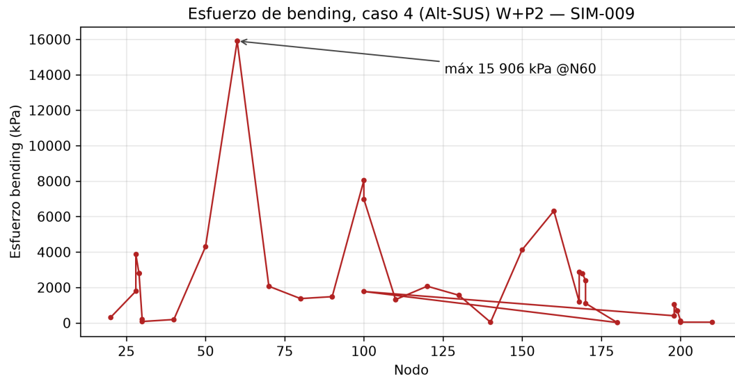
Figura 3: Perfil de esfuerzo de flexión por nodo, caso crítico 4 (Alt-SUS) W+P2. Máximo: 15 905,8 kPa en el nodo 60.
