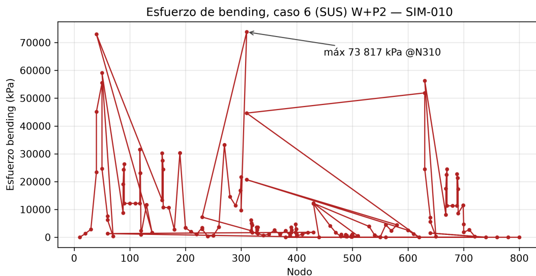
Figura 3: Perfil de esfuerzo de flexión por nodo, caso crítico 6 (SUS) W+P2. Máximo: 73 816,8 kPa en el nodo 310.
