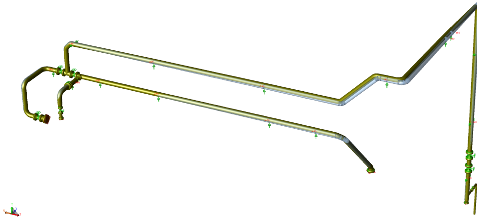
Figura 4: Configuración deformada del modelo de la línea, vista opuesta (CAESAR II, job P2603-PR-SIM-011). La geometría en gris corresponde a la posición inicial y la geometría coloreada a la posición desplazada.
