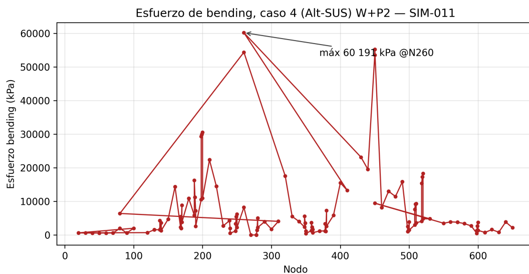
Figura 5: Perfil de esfuerzo de flexión por nodo, caso crítico 4 (Alt-SUS) W+P2. Máximo: 60 191,3 kPa en el nodo 260.
