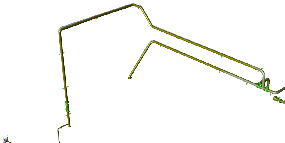
Figura 3: Configuración deformada del modelo de la línea, vista general (CAESAR II, job P2603-PR-SIM-011). La geometría en gris corresponde a la posición inicial y la geometría coloreada a la posición desplazada.
