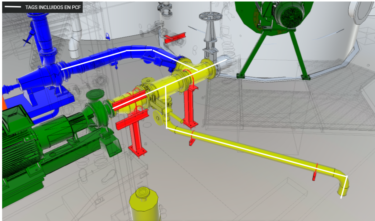
Figura 1: Isométrico de la línea de succión TK Blowtank (PCF111, AutoCAD Plant 3D 2027).
