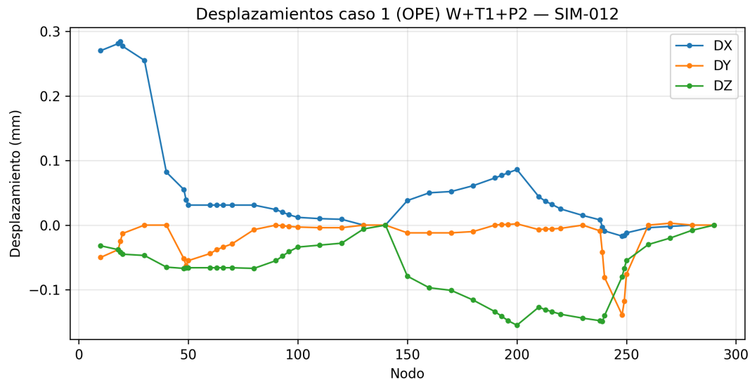
Figura 2: Perfil de desplazamientos nodales DX , DY y DZ en el caso 1 (OPE) W+T1+P2.
