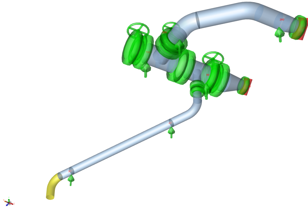
Figura 9: Modelo de CAESAR II con los soportes y restricciones de la línea, vista 2 (job P2603-PR-SIM-012).
