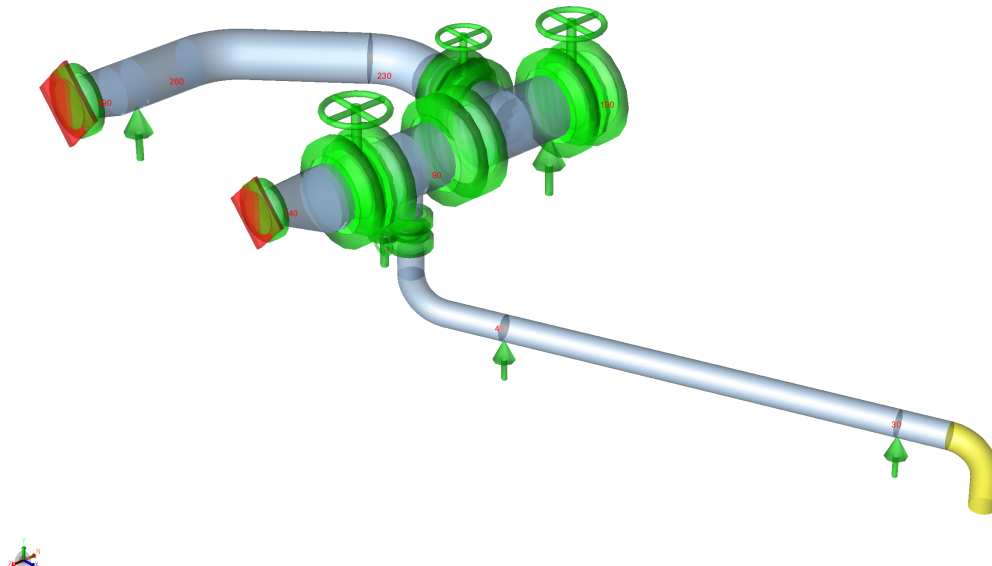
Figura 8: Modelo de CAESAR II con los soportes y restricciones de la línea, vista 1 (job P2603-PR-SIM-012).
