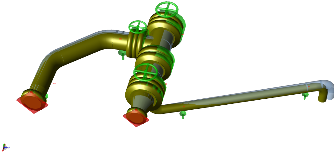
Figura 4: Vista de desplazamientos máximos del modelo, vista 2 (CAESAR II, job P2603-PR-SIM-012).
