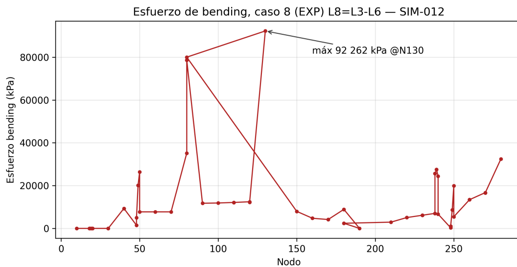
Figura 5: Perfil de esfuerzo de flexión por nodo, caso crítico 8 (EXP) L8=L3-L6. Máximo: 92 262,2 kPa en el nodo 130.
