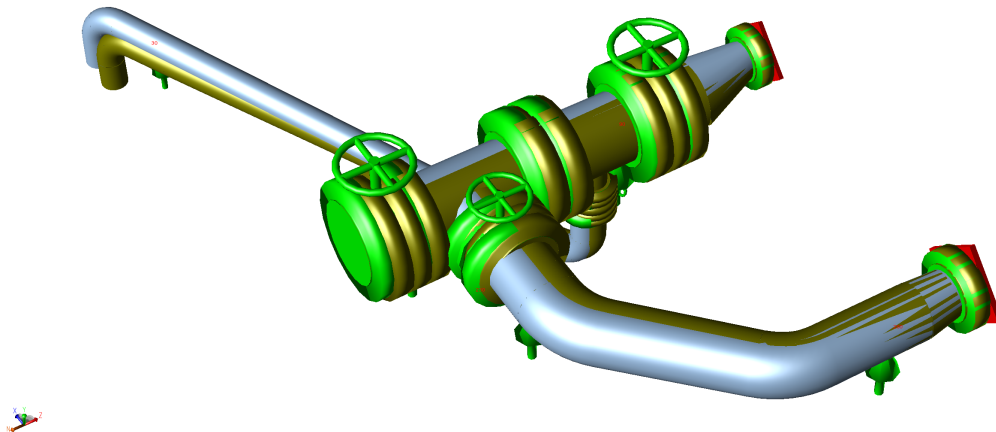
Figura 3: Vista de desplazamientos máximos del modelo, vista 1 (CAESAR II, job P2603-PR-SIM-012).
