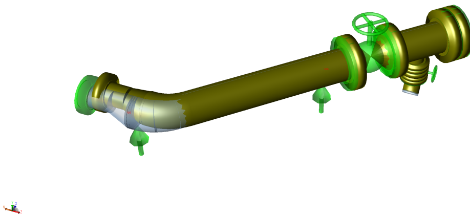
Figura 3: Configuración deformada del modelo en condición de operación, con los desplazamientos amplificados para visualización (CAESAR II, job P2603-PR-SIM-013).
