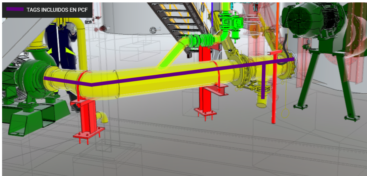
Figura 1: Vista del modelo 3D de la línea de descarga del tanque de nivelación (PCF113, AutoCAD Plant 3D 2027).
