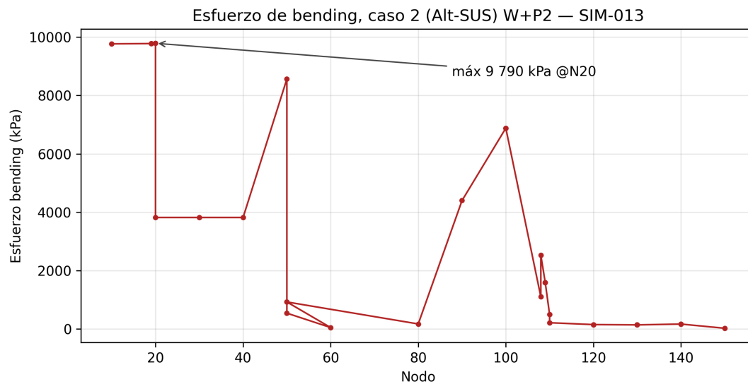
Figura 4: Perfil de esfuerzo de flexión por nodo, caso crítico 2 (Alt-SUS) W+P2. Máximo: 9789,6 kPa en el nodo 20.
