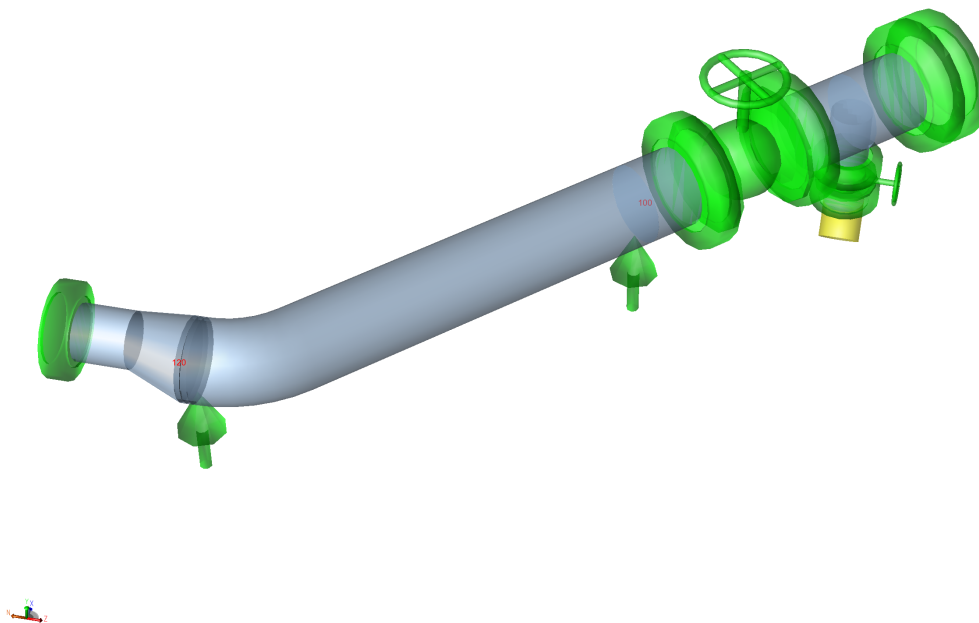
Figura 6: Modelo de CAESAR II con los soportes y restricciones de la línea (job P2603-PR-SIM-013).
