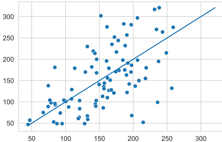
Figura 3.5: Regresión Lineal
