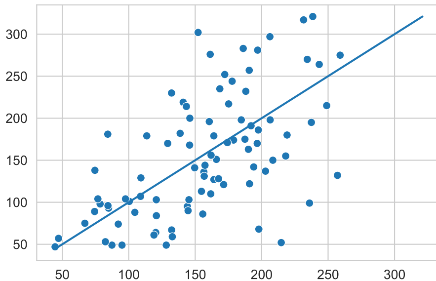
Figura 3.6: Regresión Lineal
