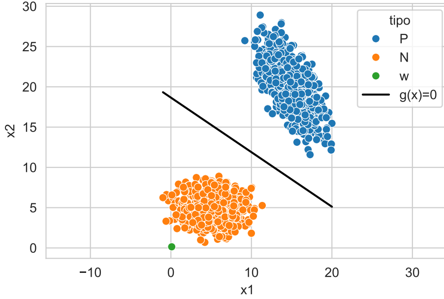
Figura 9.2: Función discriminante
