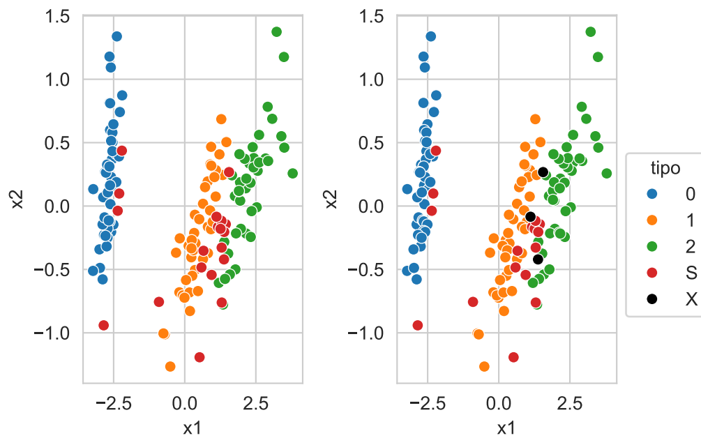
Figura 9.10: Visualización de los vectores de soporte usando PCA.
