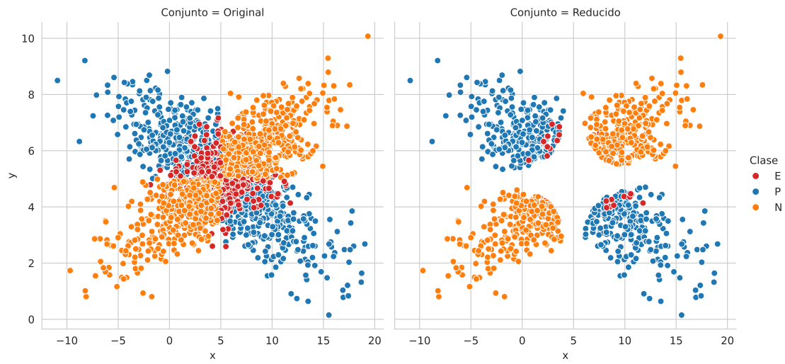
Figura 3.7: Predicción del conjunto original y el conjunto que elimina aquellos elementos que se asocian a la clase nula
