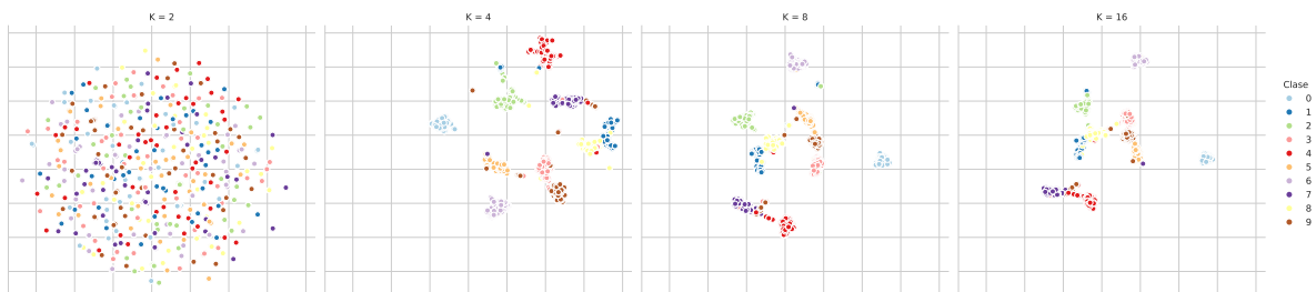
Figura 11.5: Proyección mediante UMAP del problema de Dígitos variando el número de vecinos
