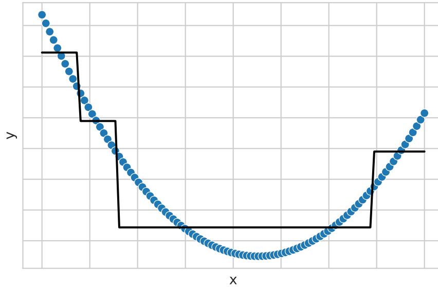
Figura 1.12: Sub-aprendizaje en un problema de regresión
