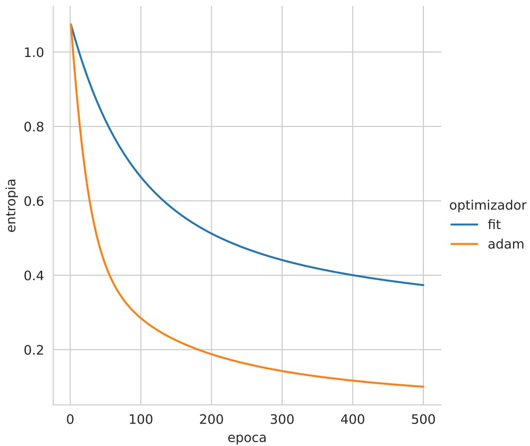
Figura 10.1: Comparación de diferentes optimizadores.
