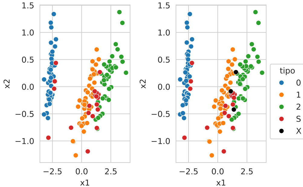
Figura 6.10: Visualización de los vectores de soporte usando PCA.
