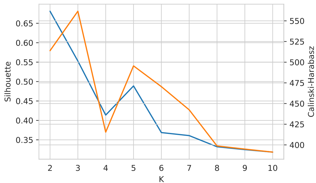
Figura 12.5: Rendimiento variando el número de grupos
