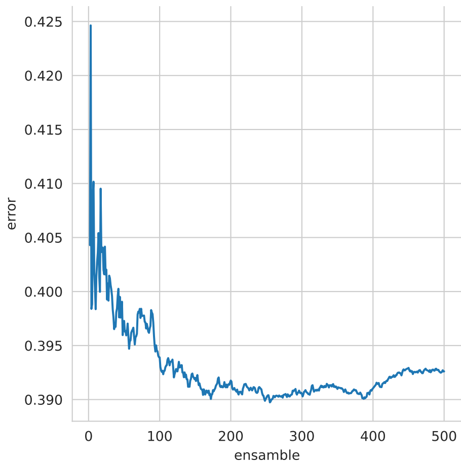
Figura 9.2: Variación del rendimiento con respecto al tamaño del ensamble ( M ).
