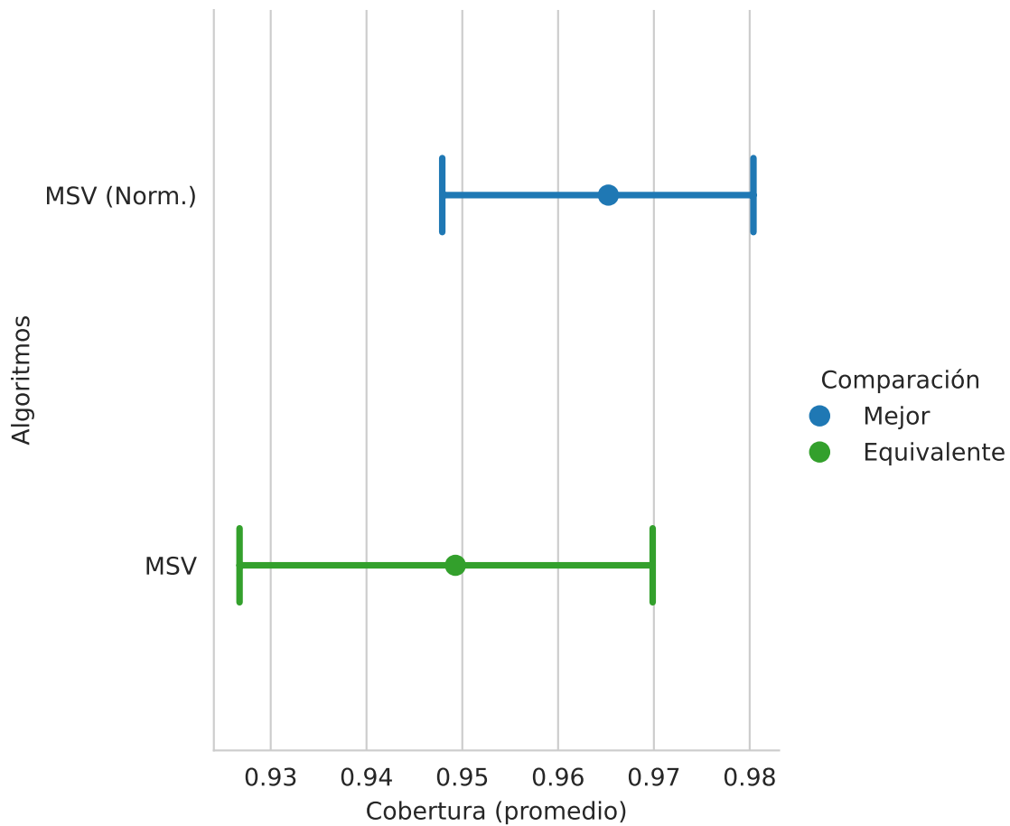
Figura 6.9: Comparación entre MSV con y sin normalización
