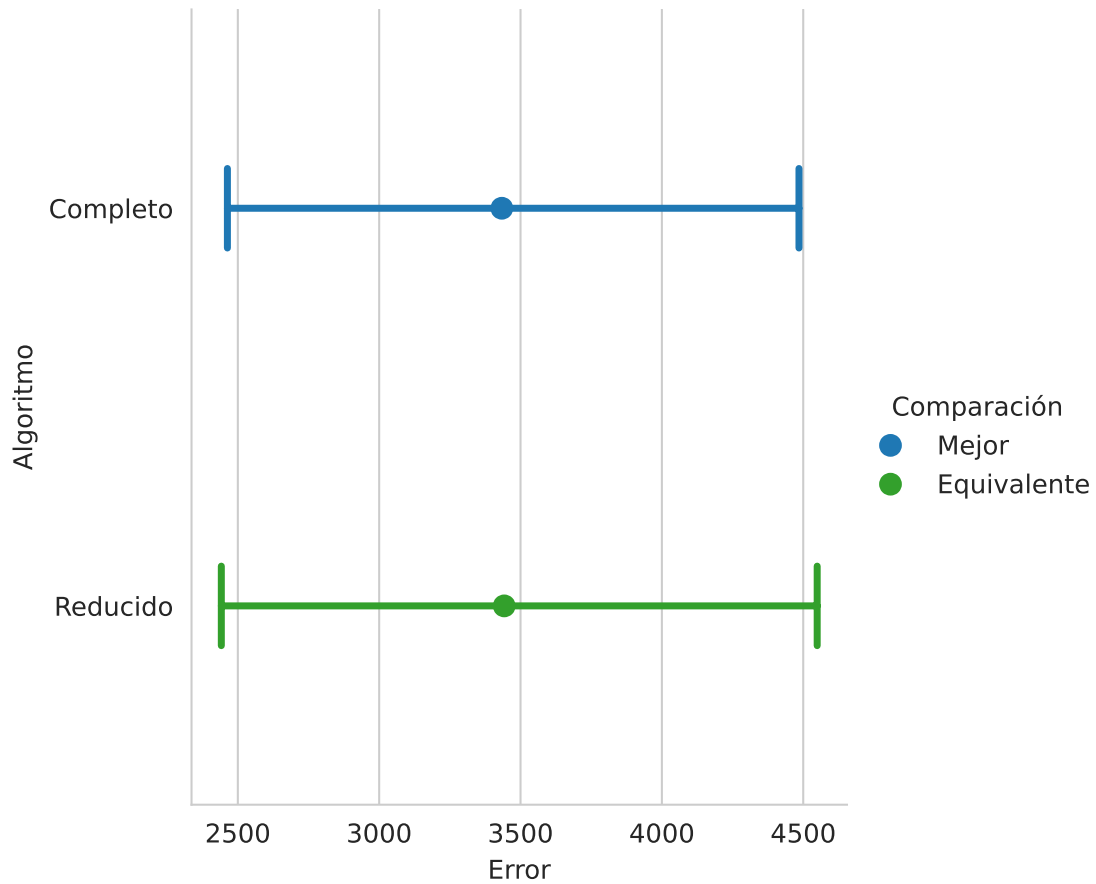
Figura 4.7: Rendimiento entre modelo con variables originales y selecc3n de variables.
