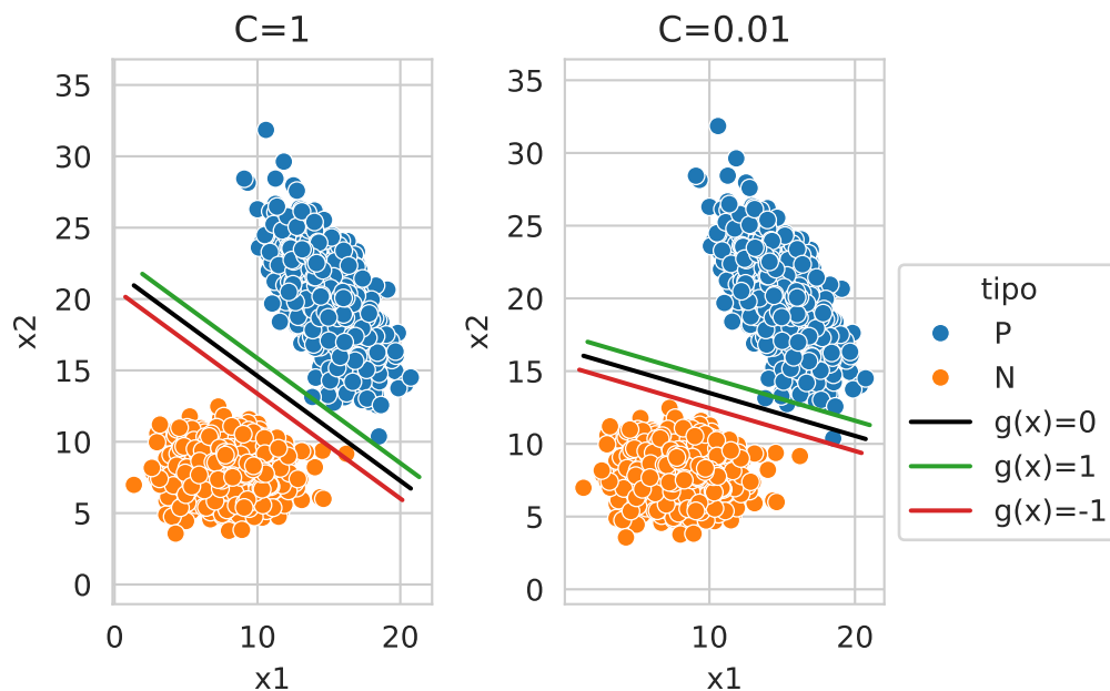
Figura 6.8: Hiperplanos para diferentes valores de C . Se observa que en C = 0.01 se clasifica incorrectamente un elemento positivo.
