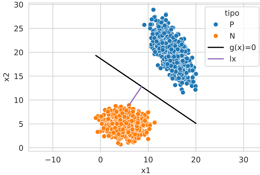
Figura 6.5: Distancia ( \ell_{\mathbf{x}} = x ) de un elemento al hiperplano
