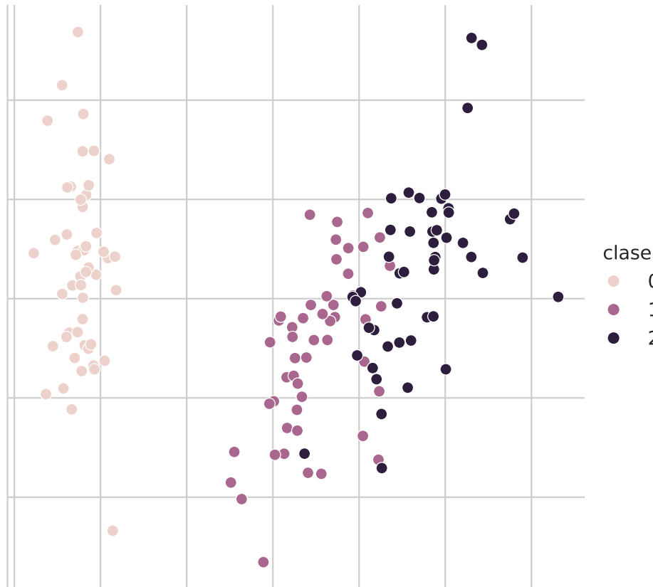
Figura 11.3: Proyección mediante PCA del problema del Iris
