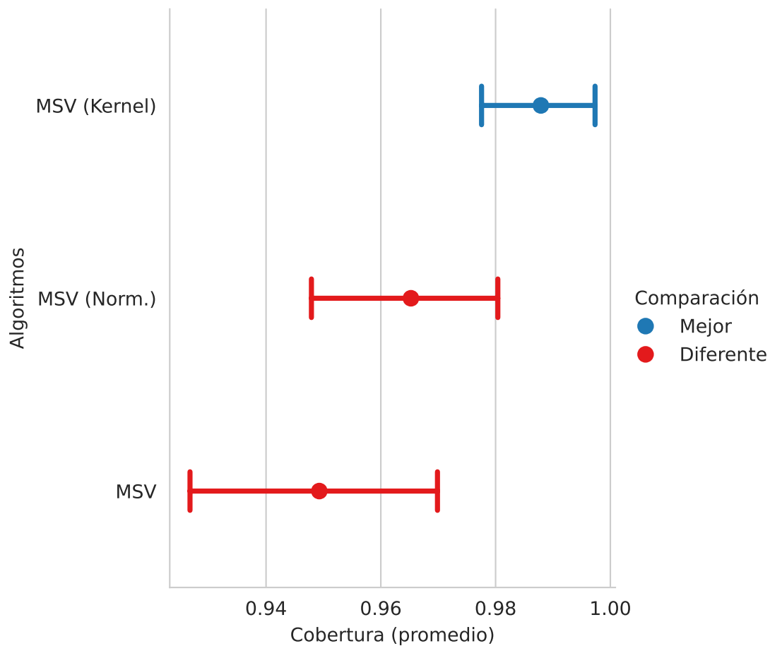
Figura 6.11: Comparación entre MSV lineales y con kernel polinomial de grado dos.
