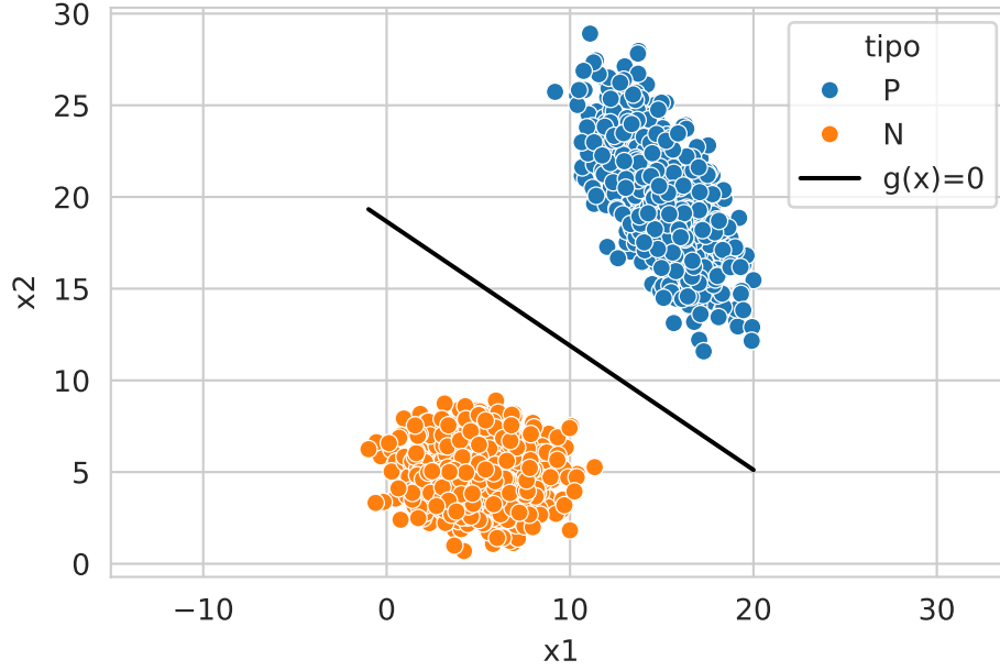
Figura 6.1: Función Discriminante
