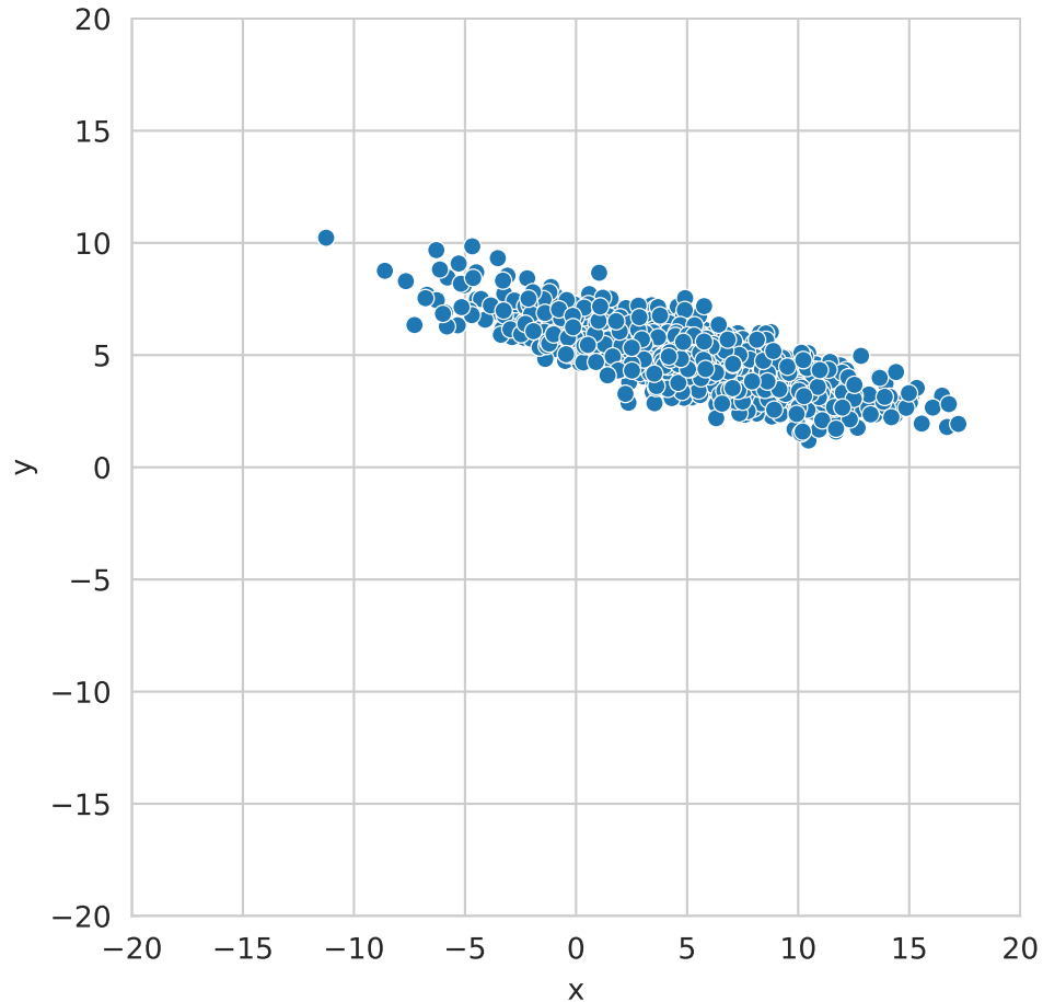
Figura 3.2: Distribución Gausiana
