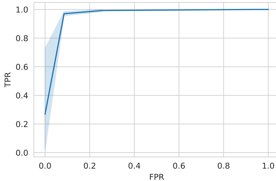
Figura 2.4: ROC
