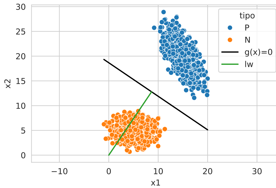
Figura 6.3: Visualizando que \mathbf{w} y la función discriminante son ortogonales.
