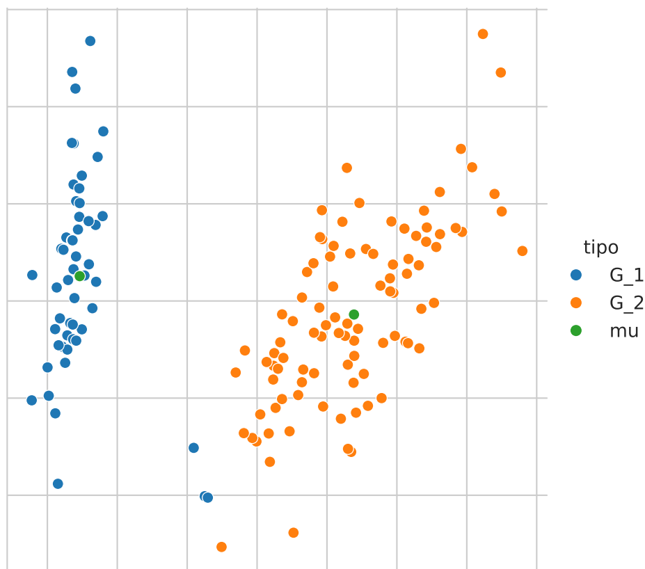
Figura 12.3: Proyección de k-means usando dos grupos
