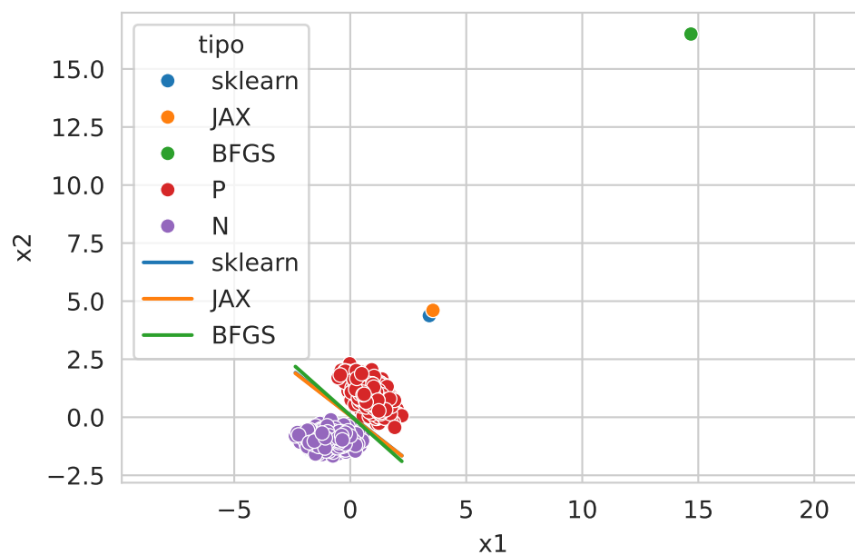
Figura 7.4: Comparación de modelos lineales con diferentes optimizadores
