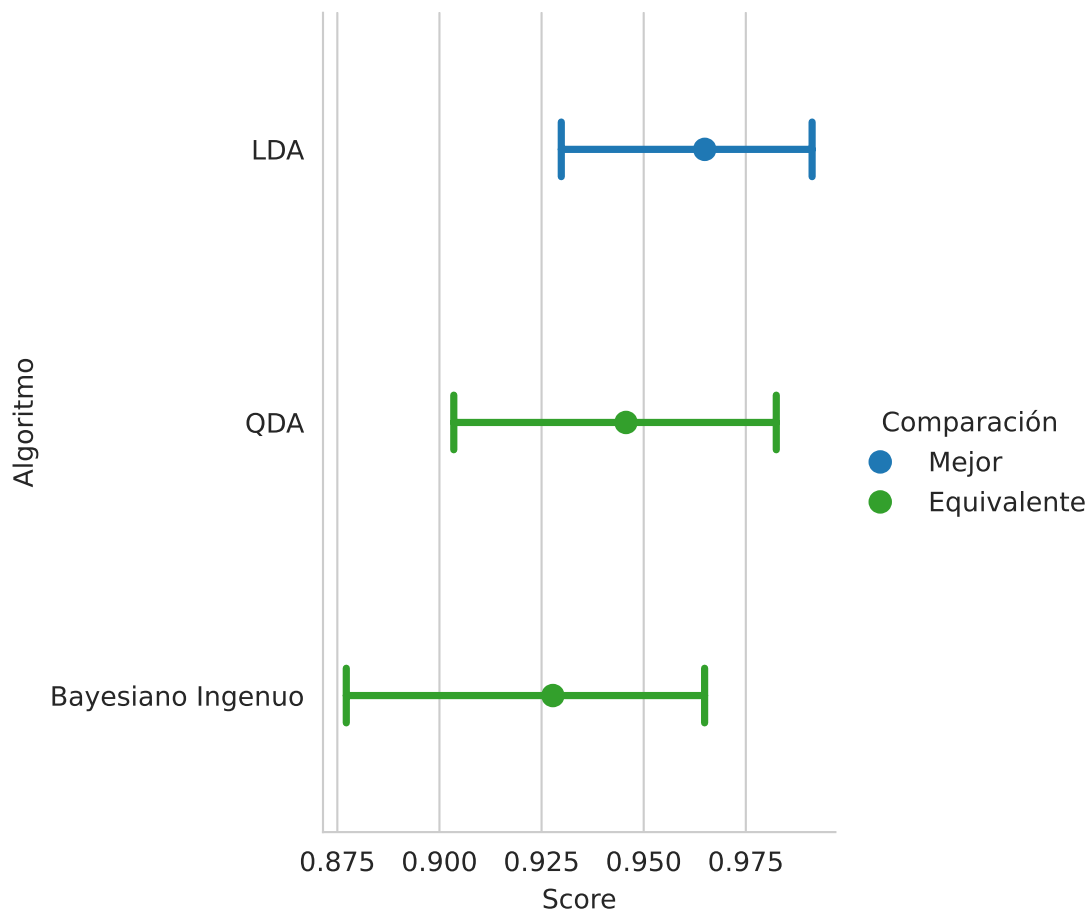
Figura 4.5: Rendimiento entre QDA y Bayesiano Ingenuo.
