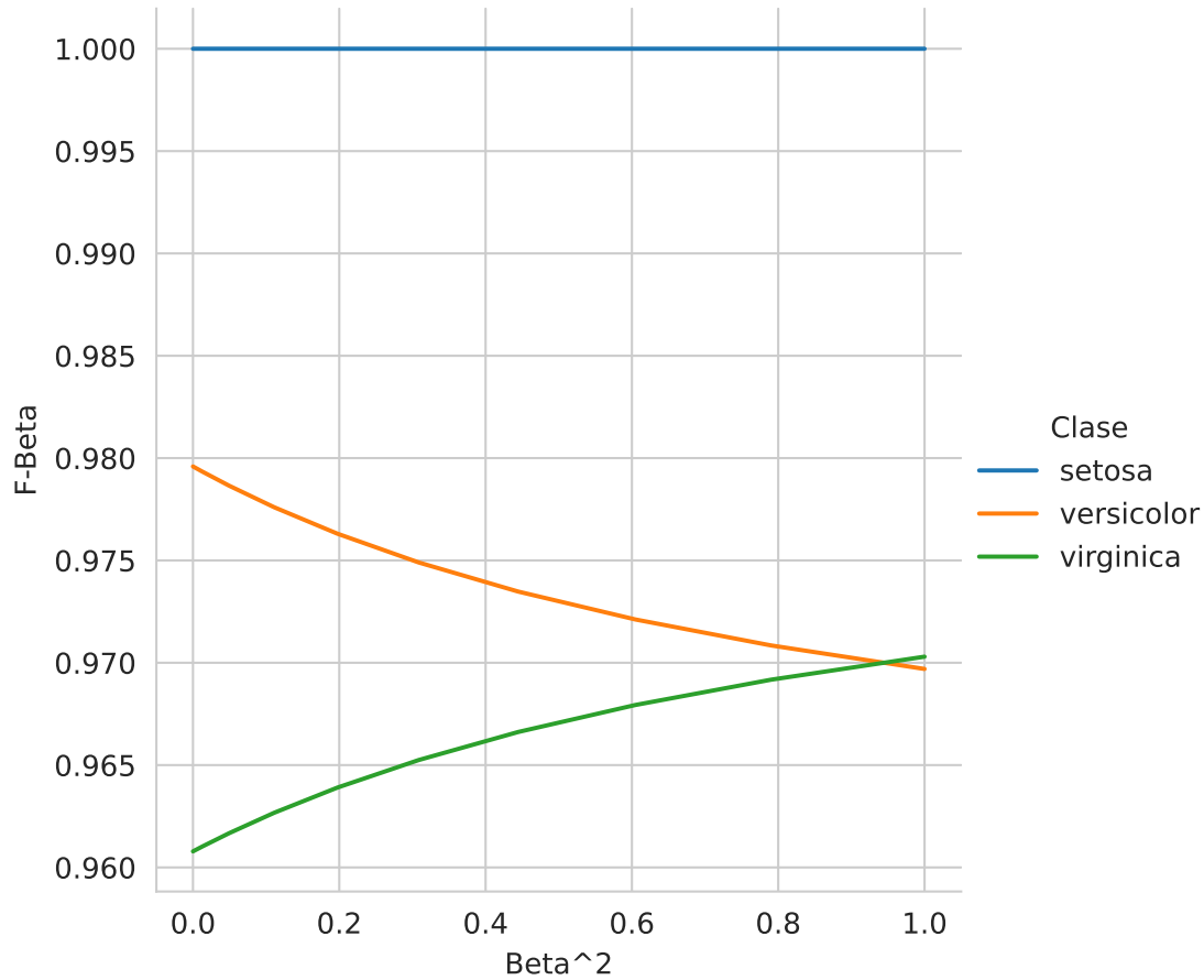
Figura 2.2: Rendimiento de un Clasificador Bayesiano Ingenuo en el problema del Iris estimado mediante una validación cruzada estratificada.
