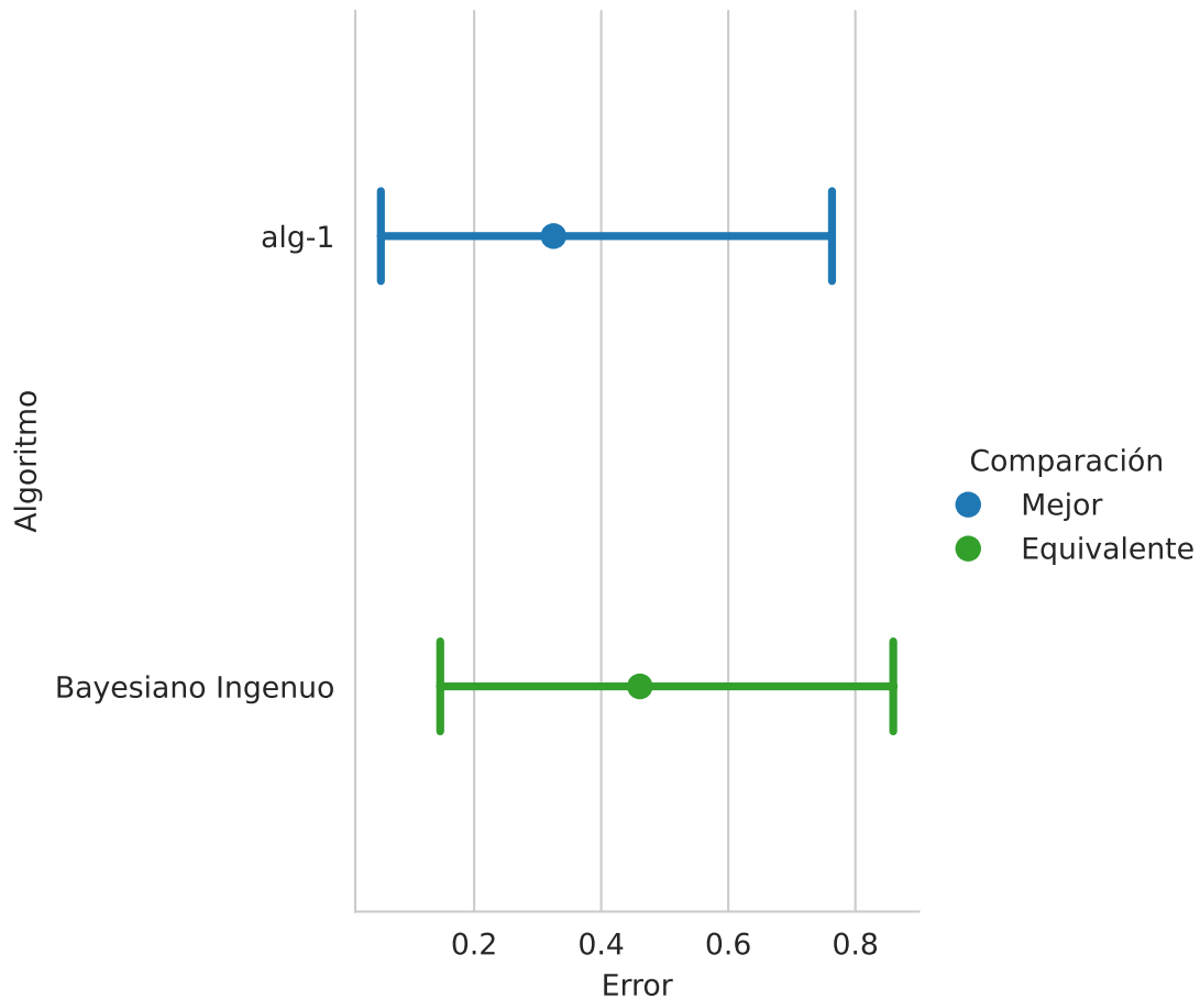
Figura 2.3: Rendimiento usando entropía cruzada entre alg-1 (Analizador Discriminante Cuadrático) y Bayes Ingenuo
