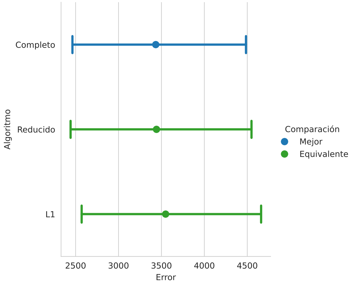
Figura 4.8: Rendimiento entre modelo con variables originales, con la norma L_1 y selección de variables.
