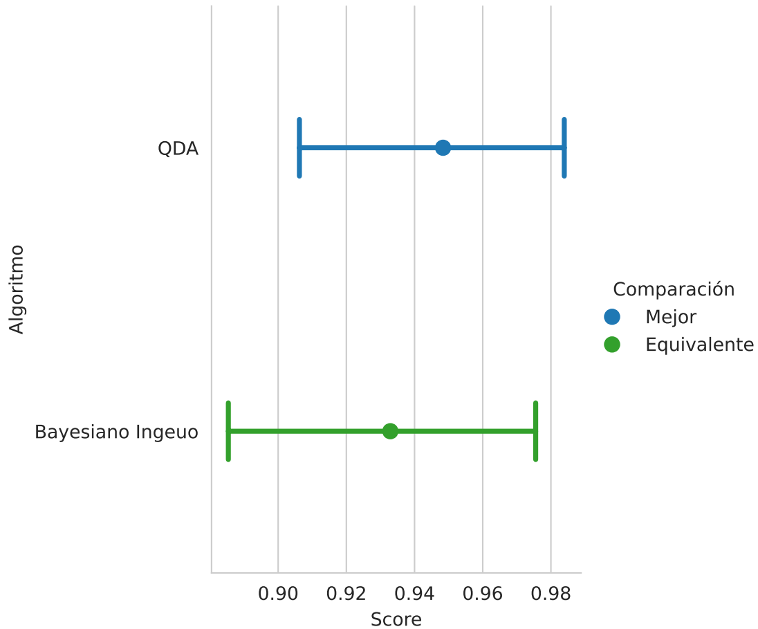
Figura 2.5: Comparación de la cobertura en el conjunto de validación
