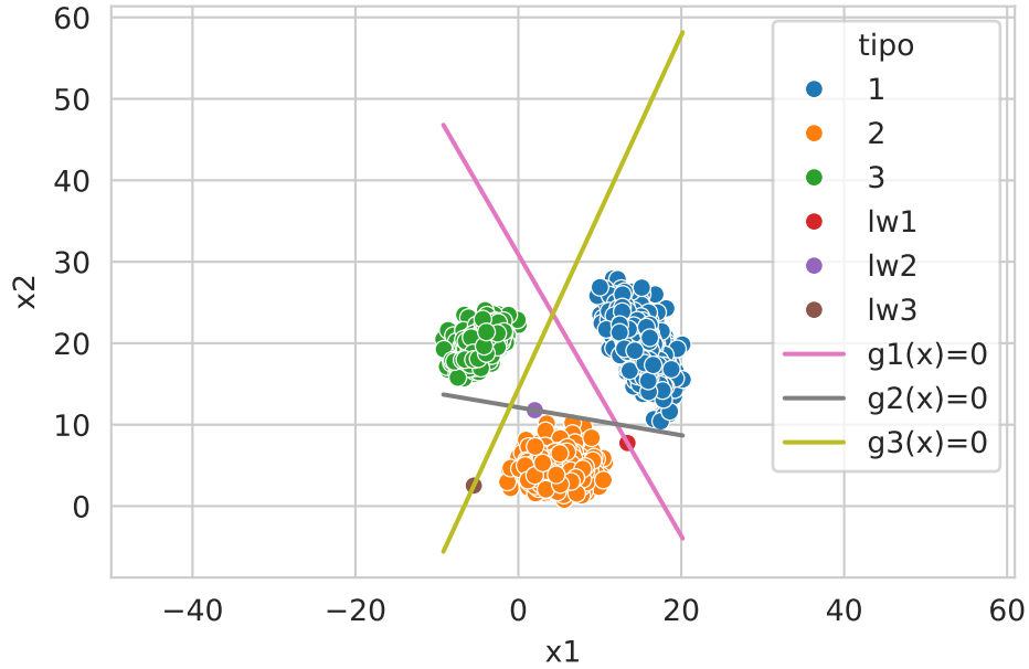
Figura 6.6: Problema multiclase
