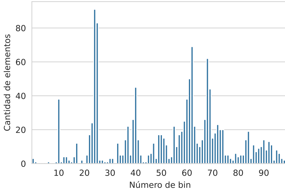
Figura 5.1: Histograma
