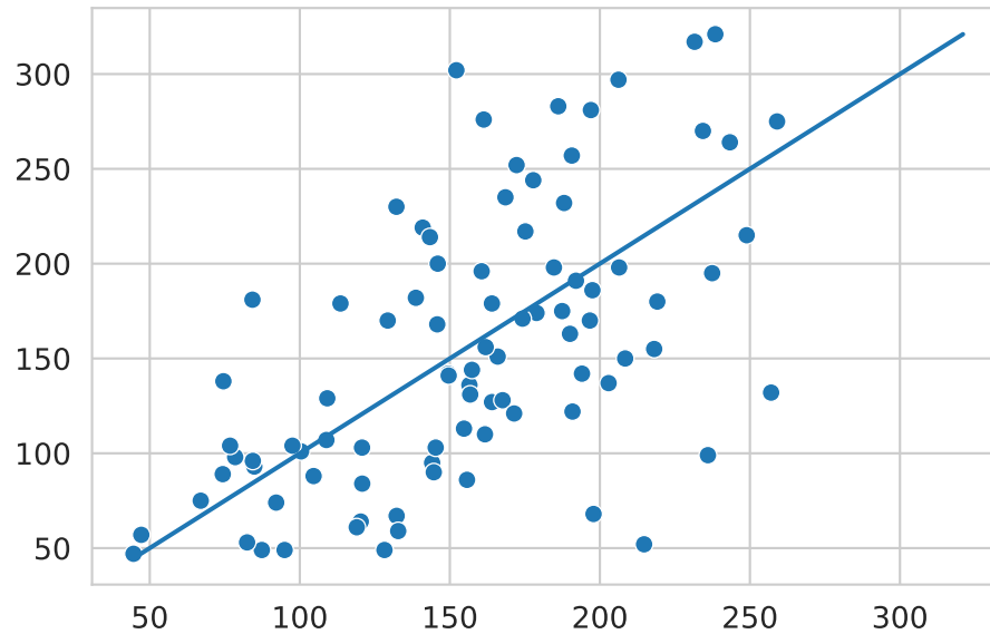
Figura 4.6: Regresión Lineal
