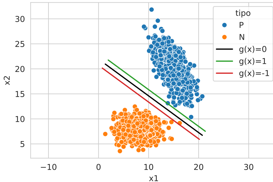
Figura 6.7: Hiperplanos
