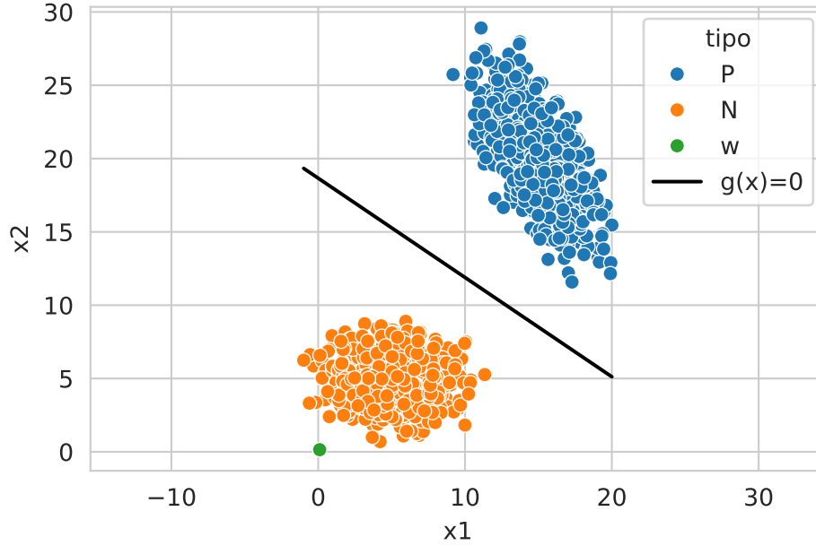
Figura 6.2: Función discriminante
