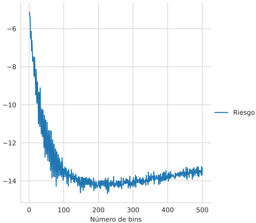
Figura 5.2: Riesgo
