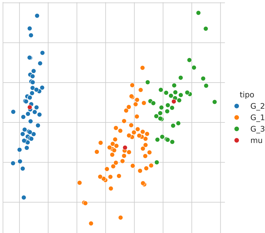
Figura 12.4: Proyección de k-means usando tres grupos
