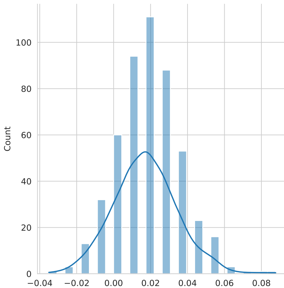
Figura 4.3: Diferencia entre Clasificadores Bayesianos
