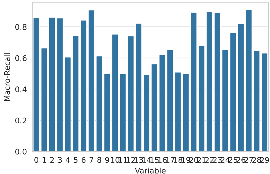
Figura 11.1: Rendimiento de las variables en la primera iteración del selección hacia adelante
