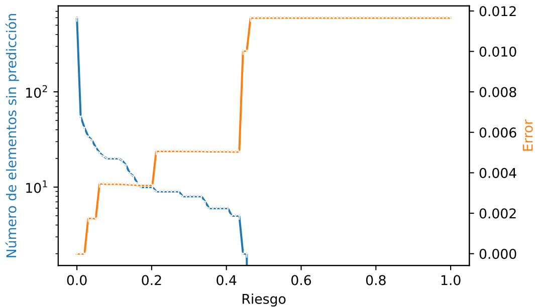
Figura 4.1: Variación del número de elementos que seleccionan la acción nula y el error en el conjunto de prueba respecto al riesgo
