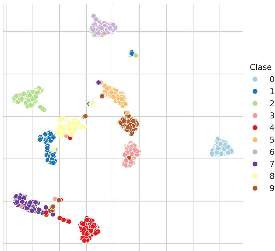
Figura 11.6: Proyección mediante UMAP del problema de dígitos con ocho vecinos
