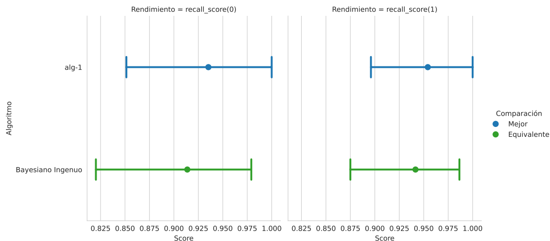
Figura 2.1: Rendimiento entre alg-1 (Analizador Discriminante Cuadrático) y Bayes Ingenuo
