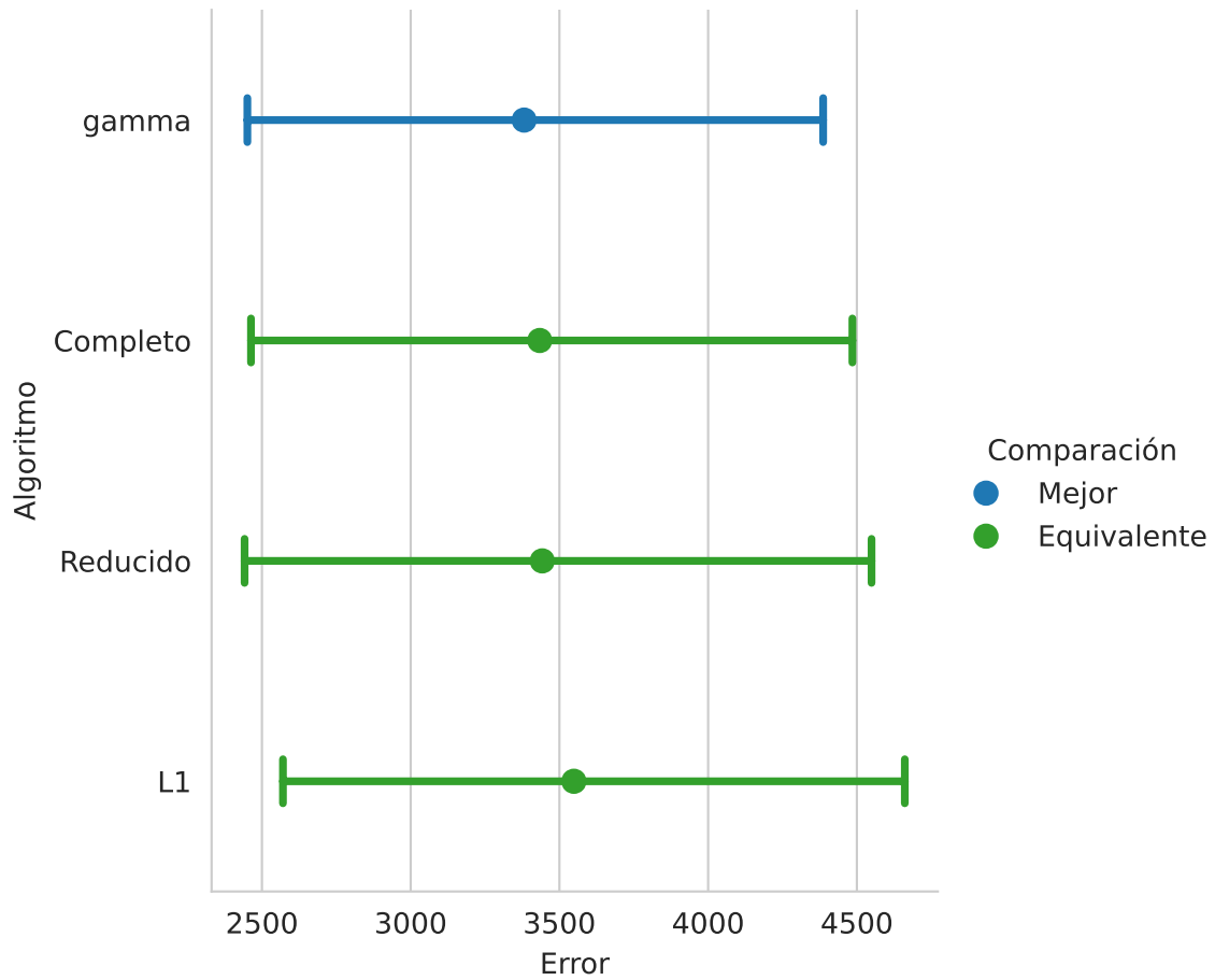
Figura 4.9: Rendimiento entre diferentes modelos.
