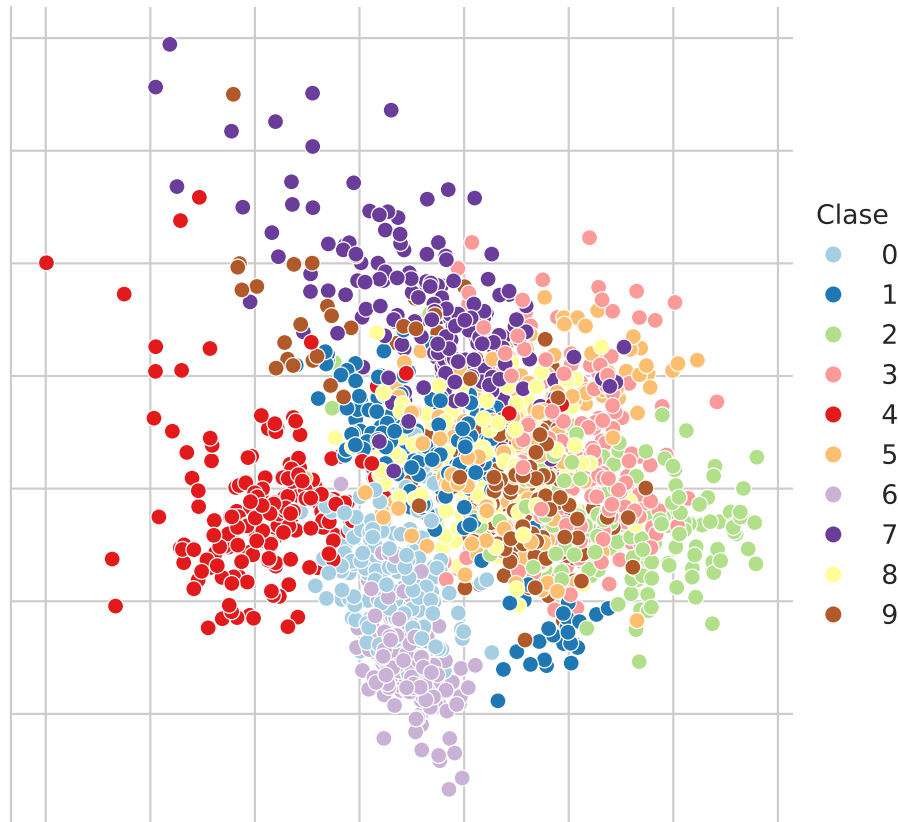
Figura 11.4: Proyección mediante PCA del problema de Dígitos
