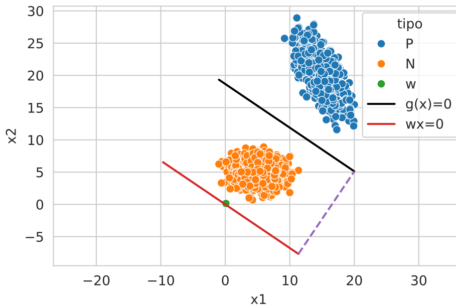
Figura 6.4: Geometría de la función discriminante.
