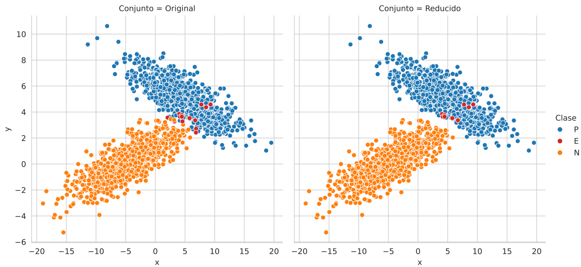
Figura 3.6: Predicción del conjunto original y el conjunto que elimina aquellos elementos que se asocian a la clase nula
