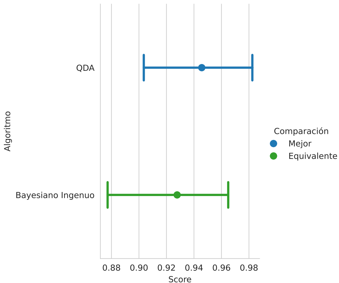
Figura 4.4: Rendimiento entre QDA y Bayesiano Ingenuo.
