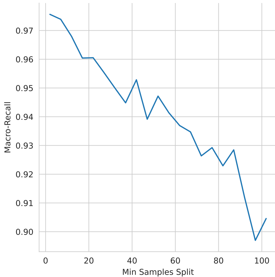
Figura 9.3: Cambio del rendimiento cuando el parámetro que controla el número de muestras para realizar la partición (i.e., min_samples_split ) varía.
