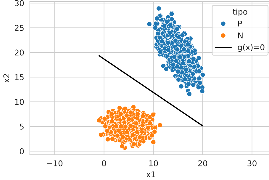
Figura 6.1: Función Discriminante
