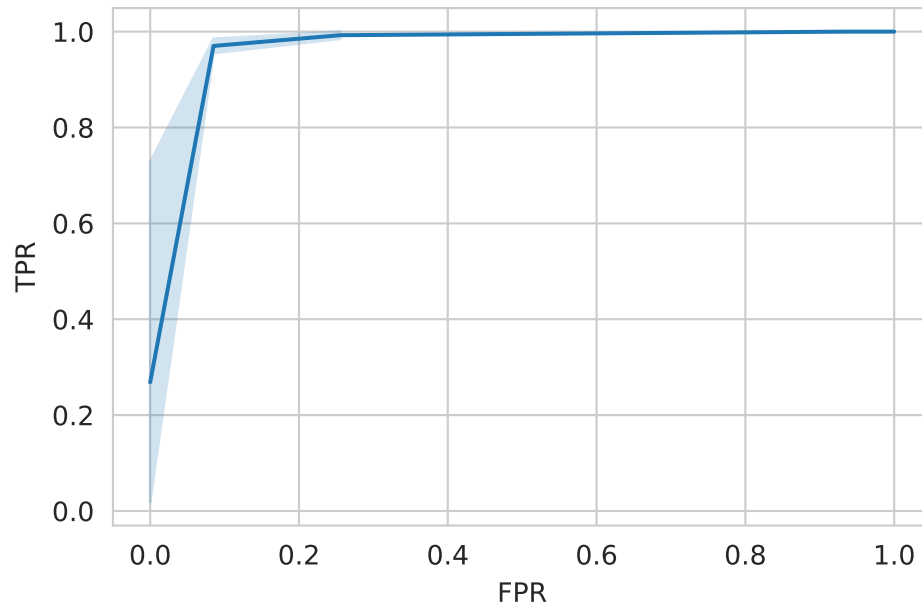
Figura 2.4: ROC
