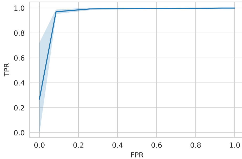
Figura 4.4: ROC
