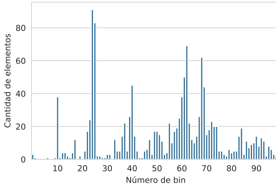
Figura 7.1: Histograma
