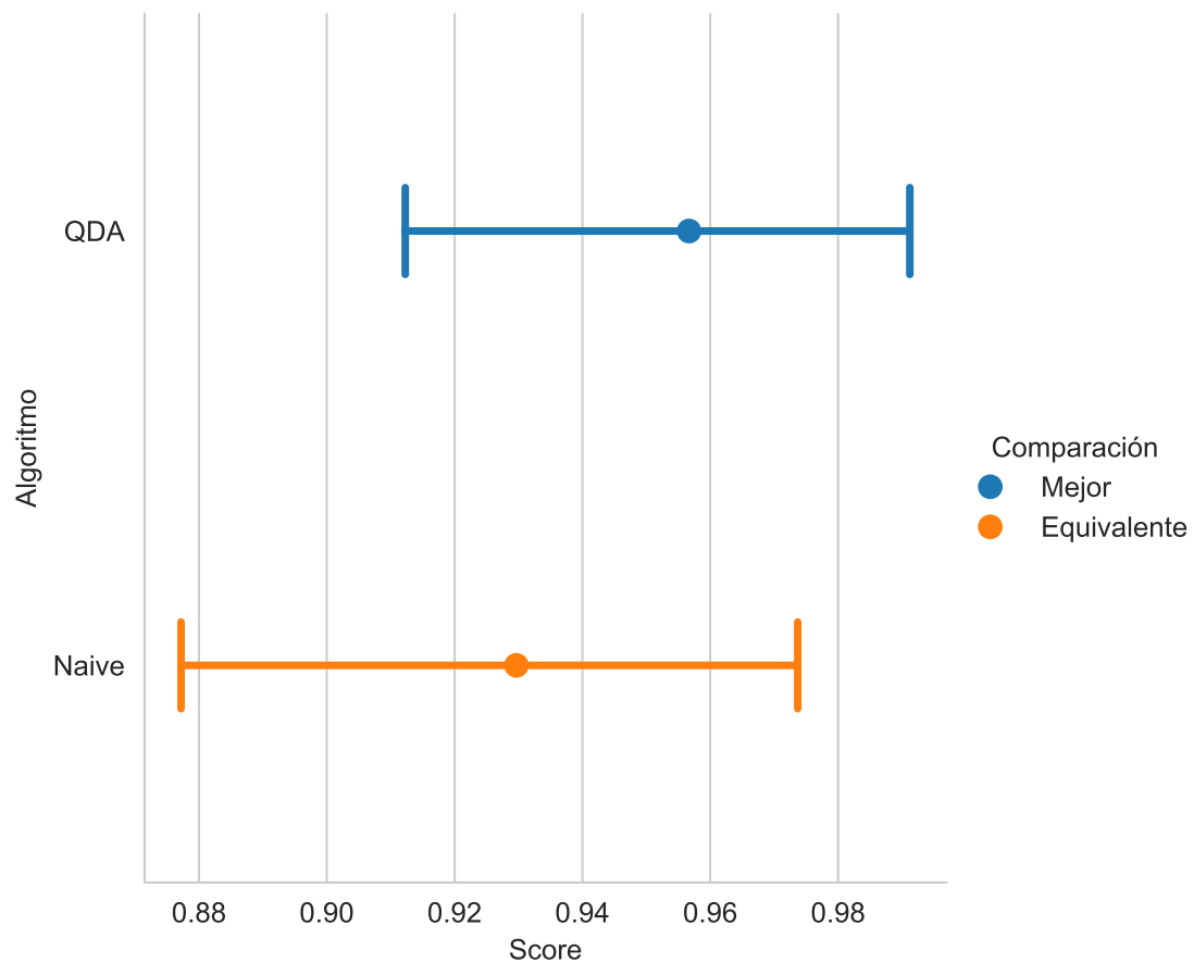
Figura 3.4: Rendimiento entre QDA y Naive Bayes.
