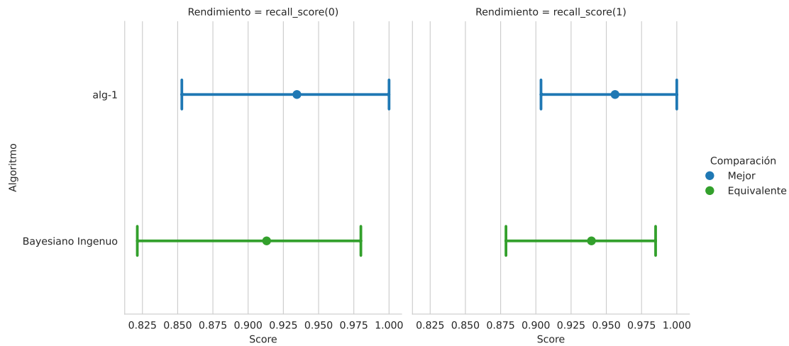
Figura 4.1: Rendimiento entre alg-1 (Analizador Discriminante Cuadrático) y Bayes Ingueno
