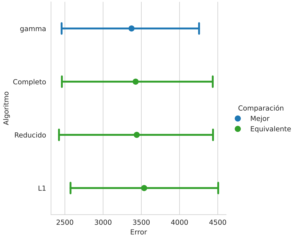
Figura 3.9: Rendimiento entre diferentes modelos.
