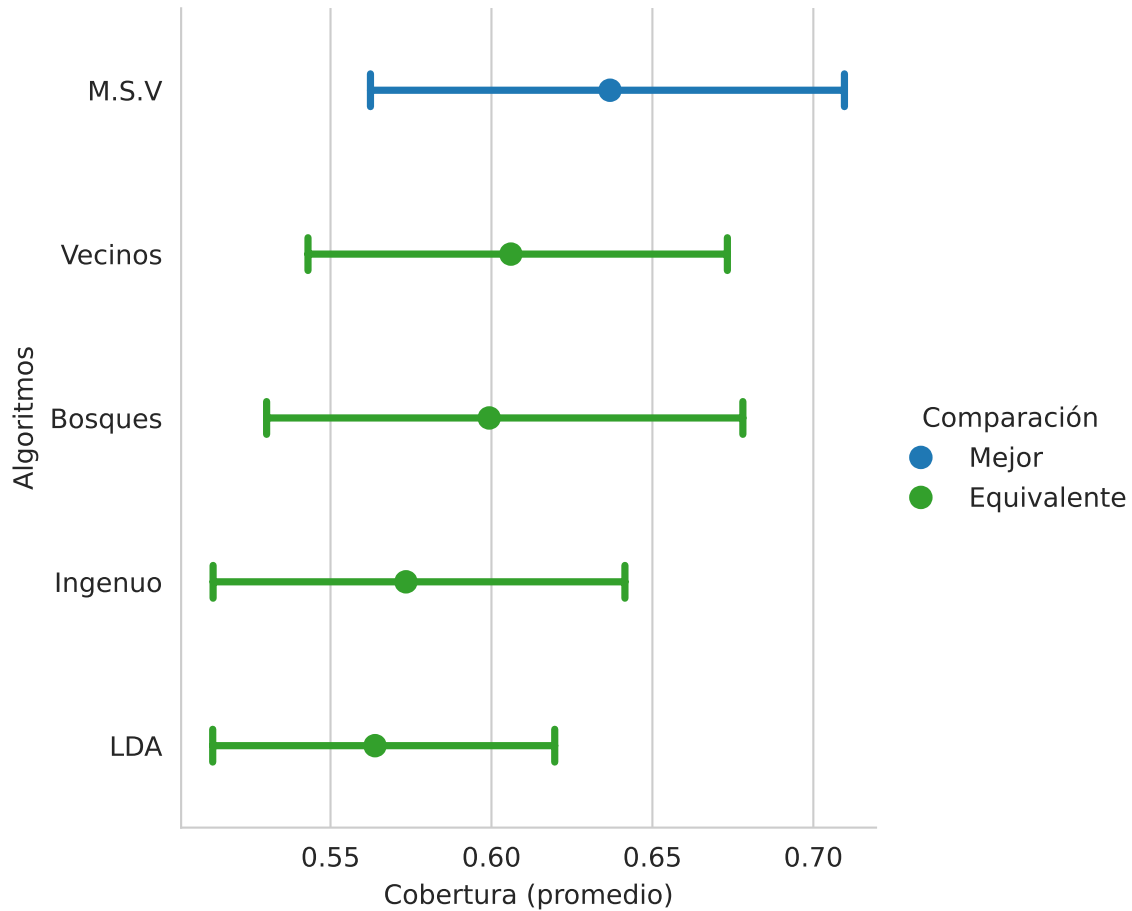
Figura 1.10: Comparación del rendimiento de algoritmos de clasificación en el conjunto de prueba.
