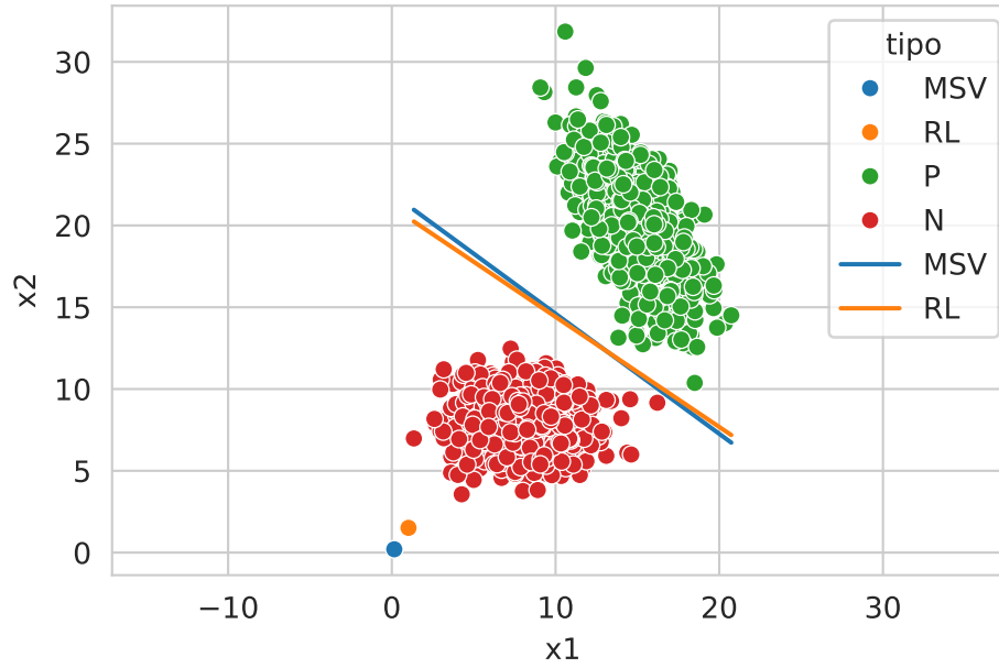
Figura 9.12: Comparación de dos métodos lineales
