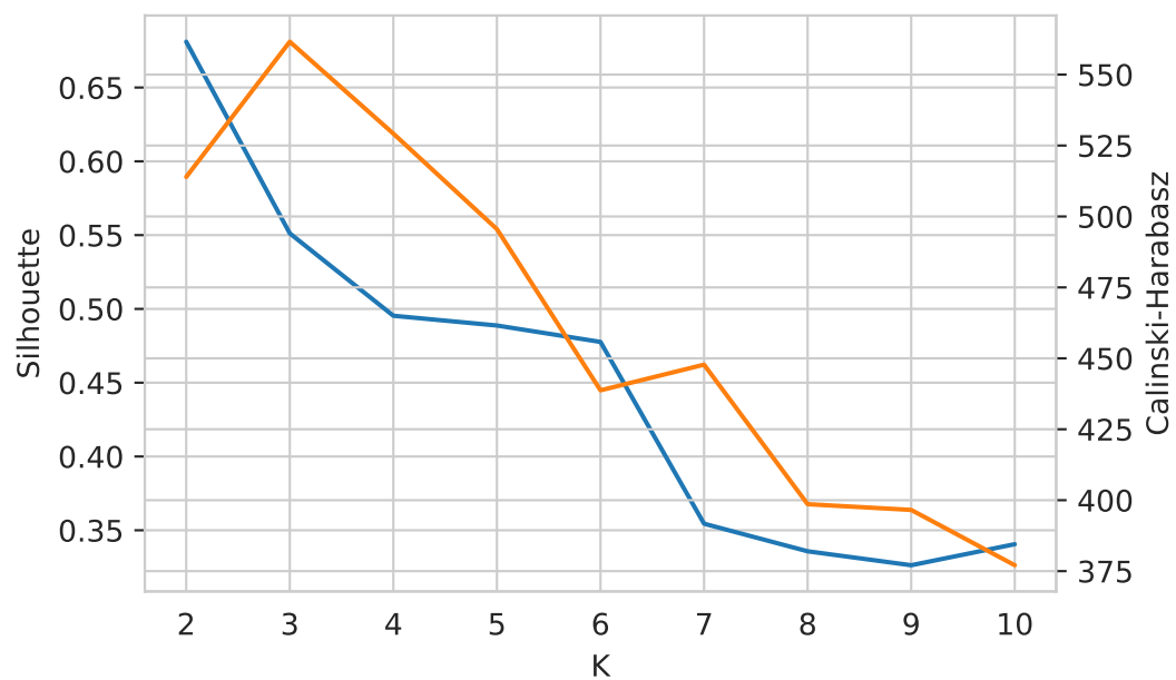
Figura 6.5: Rendimiento variando el número de grupos
