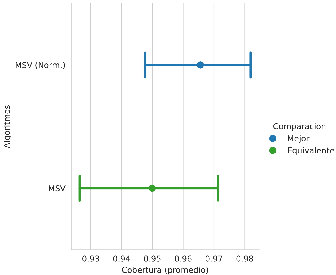
Figura 9.9: Comparación entre MSV con y sin normalización
