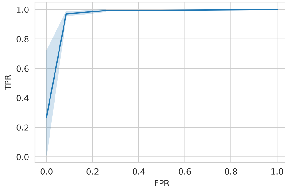
Figura 4.4: ROC
