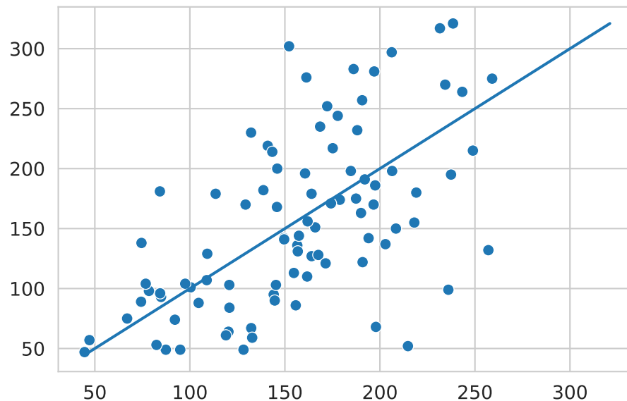
Figura 3.6: Regresión Lineal
