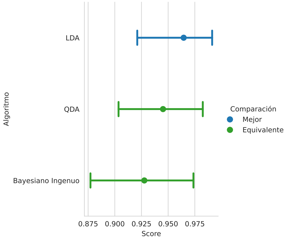
Figura 3.5: Rendimiento entre QDA y Bayesiano Ingenuo.
