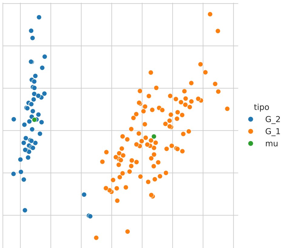
Figura 6.3: Proyección de k-means usando dos grupos
