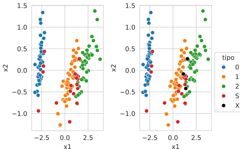
Figura 9.10: Visualización de los vectores de soporte usando PCA.
