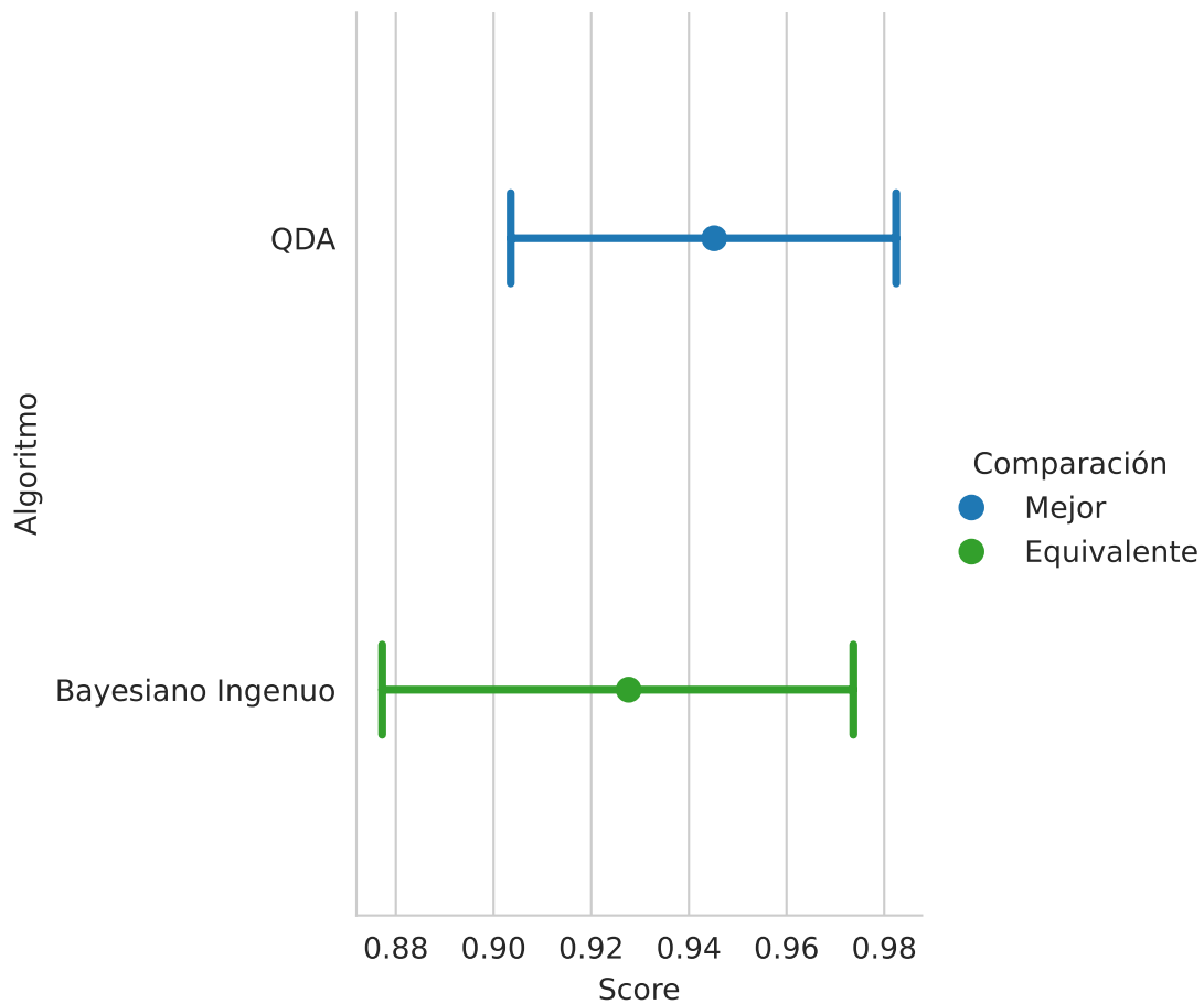
Figura 3.4: Rendimiento entre QDA y Bayesiano Ingenuo.
