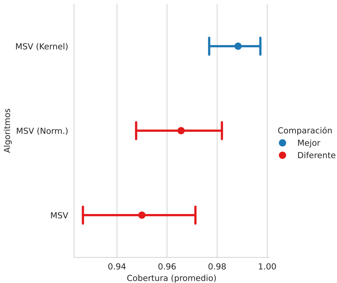
Figura 9.11: Comparación entre MSV lineales y con kernel polinomial de grado dos.
