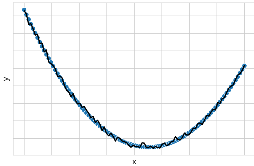
Figura 1.11: Sobre-aprendizaje en un problema de regresión
