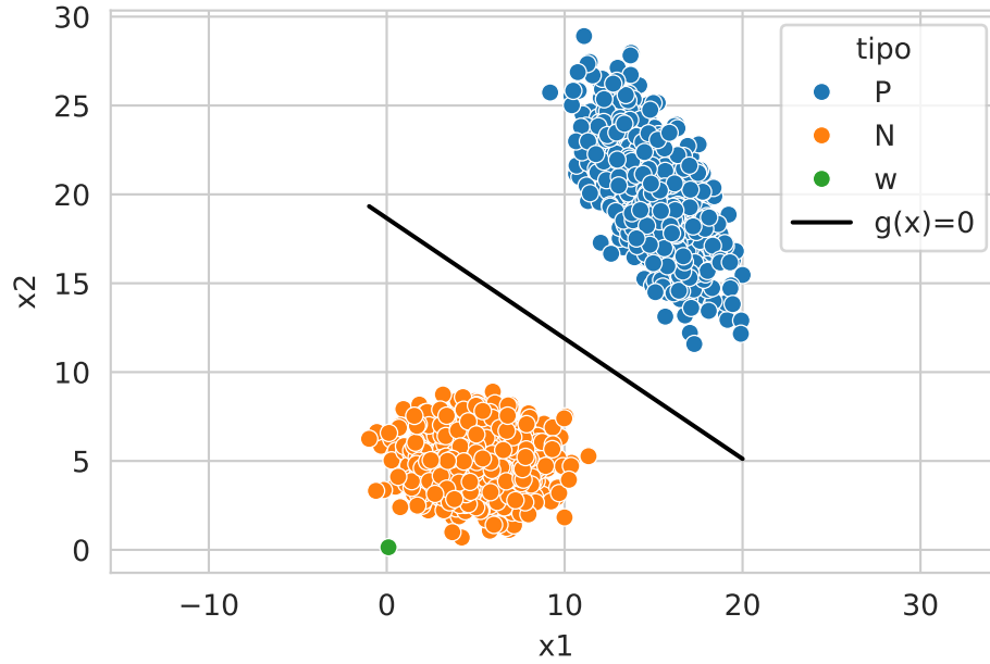
Figura 9.2: Función discriminante
