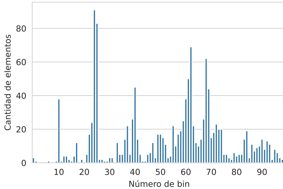
Figura 7.1: Histograma
