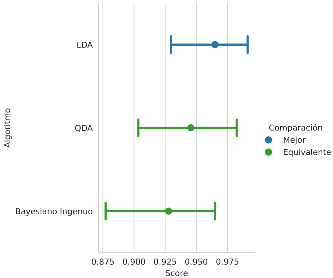
Figura 4.5: Rendimiento entre QDA y Bayesiano Ingenuo.
