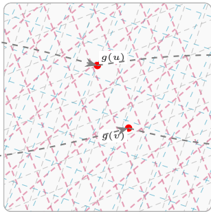
Funciones LSH
